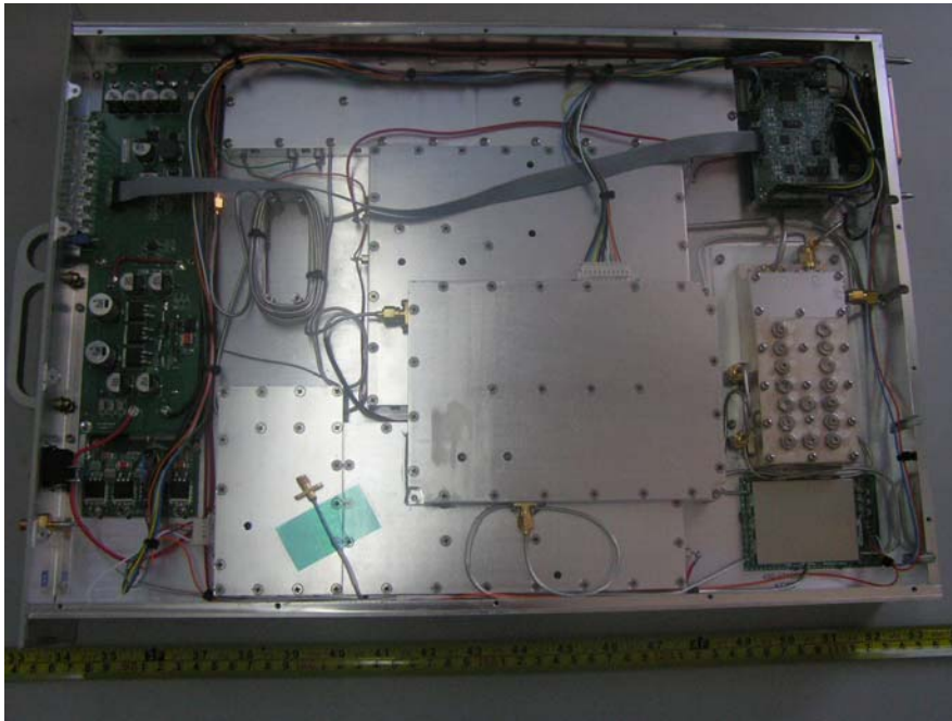
LPA1900MHz Remec-4
