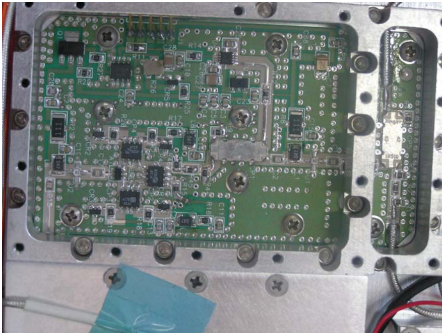
LPA1900MHz Remec-9
