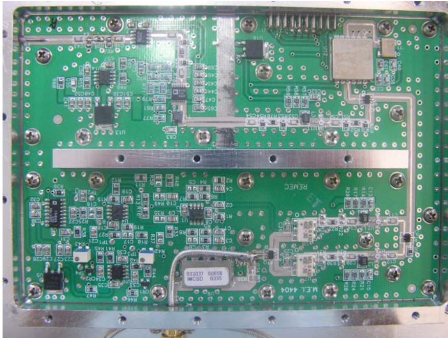
LPA1900MHz Remec-9
