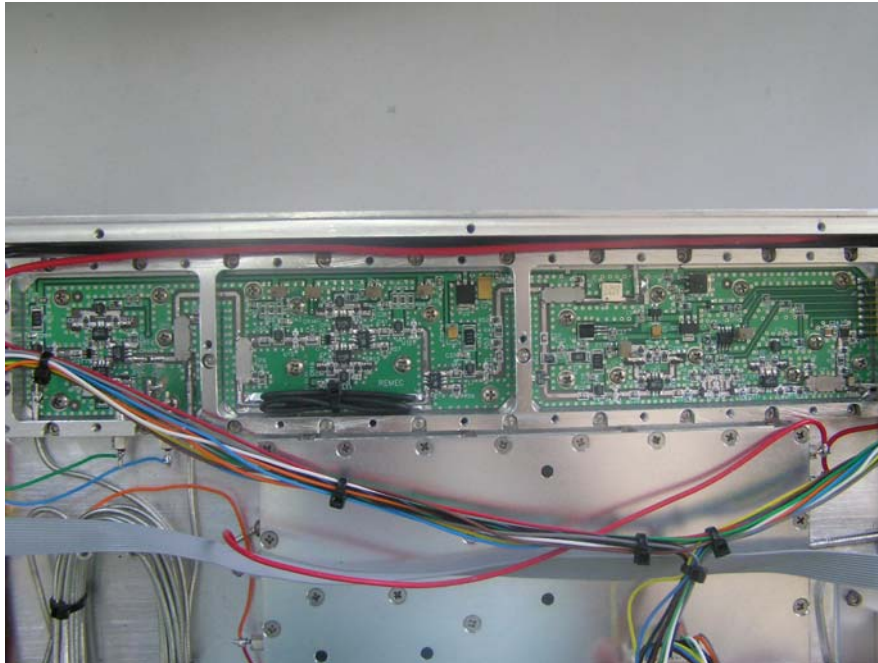
LPA1900MHz Remec-10
