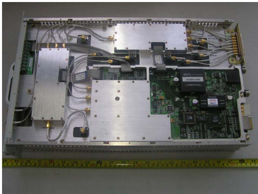
RFE1900MHz Allrizon-4
