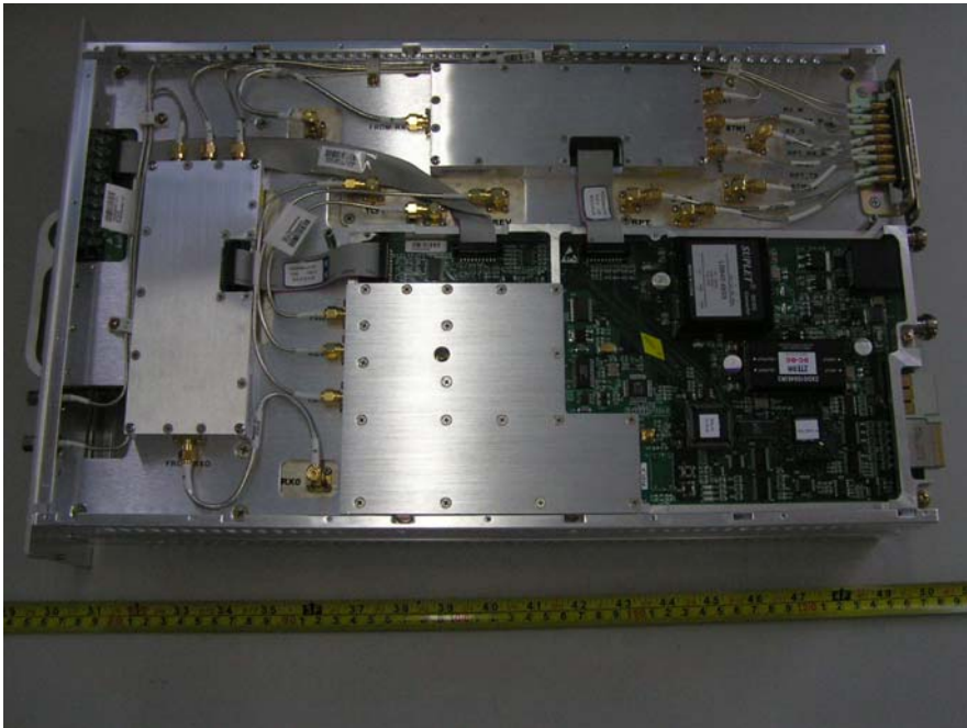
RFE1900MHz M.B-1
