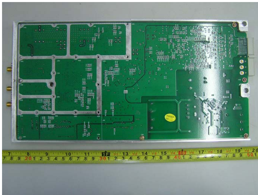
RFE1900MHz M.B-4
