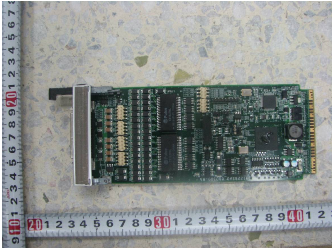
Front view of SA board
