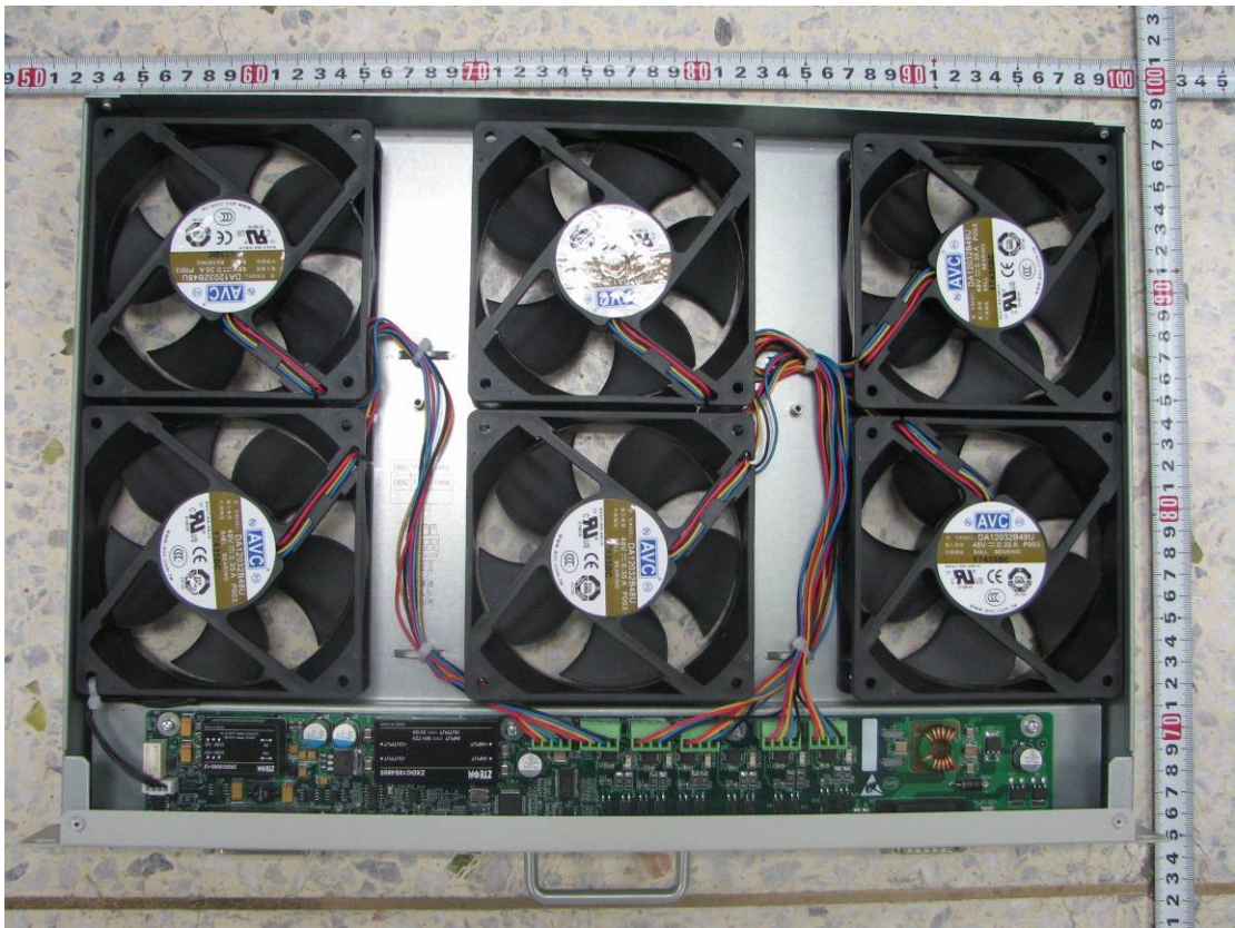
Fan module (front view)
