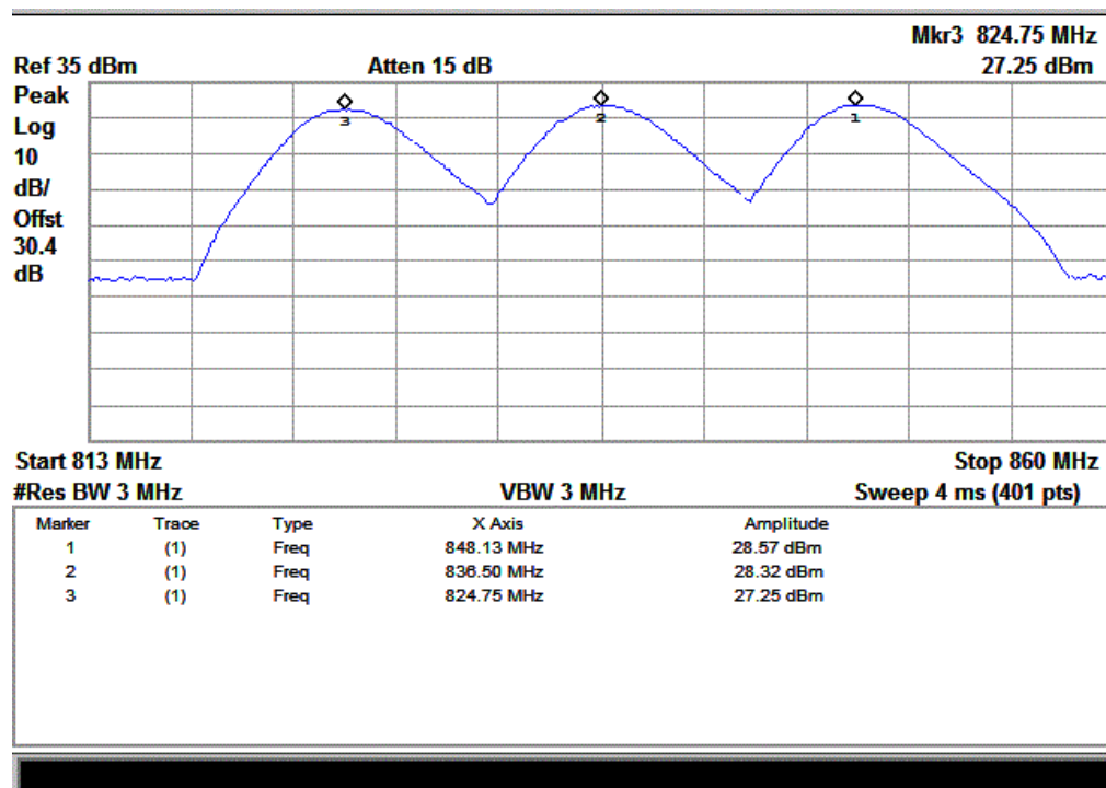
(Plot A: CDMA 800MHz Channel = 1013, 384, 777)
