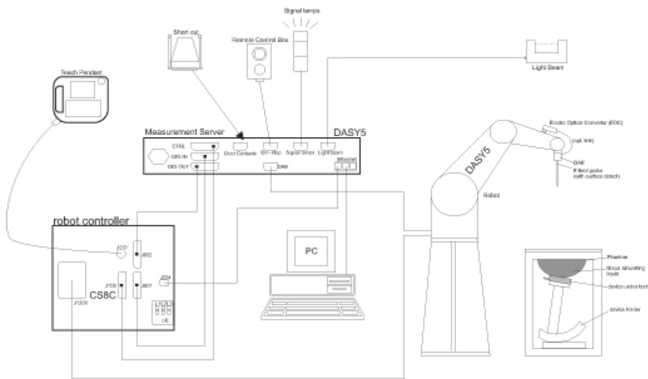
Fig. 5.1 DASY5 System
