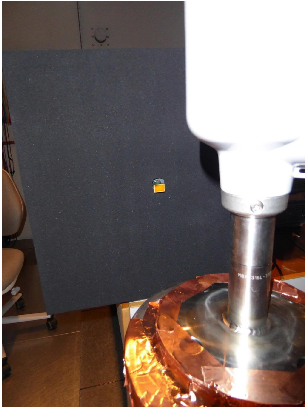
Test setup (>40 GHz)
