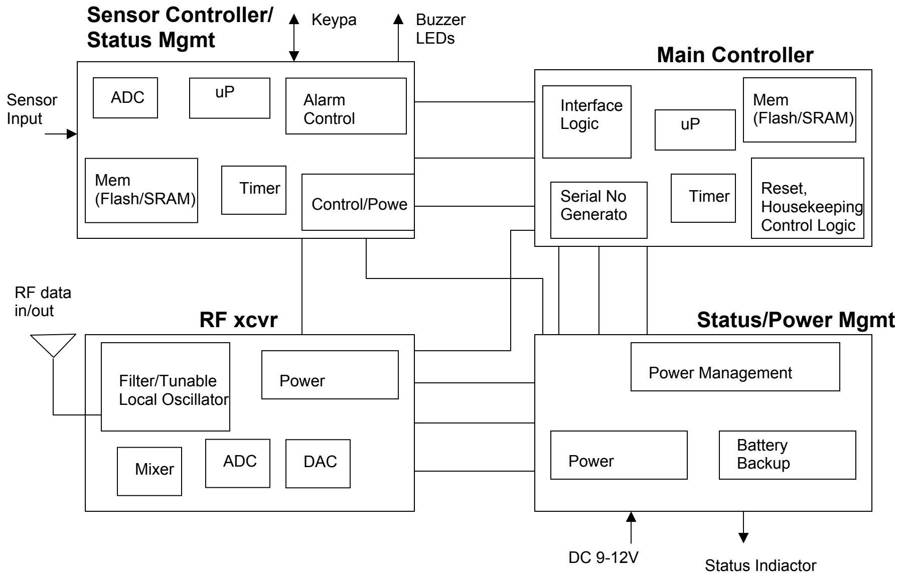
CP Block Diagram
