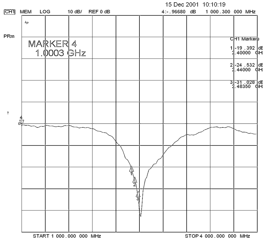
Fig 1. Returnloss
