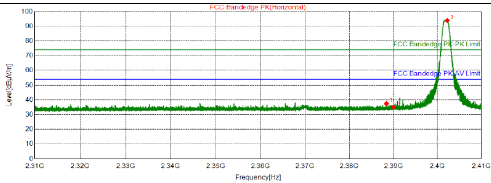
BLE_2402_Ant1/ Horizontal
