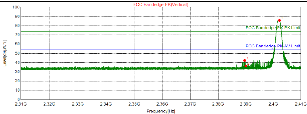
BLE_2402_Ant1/ Vertical
