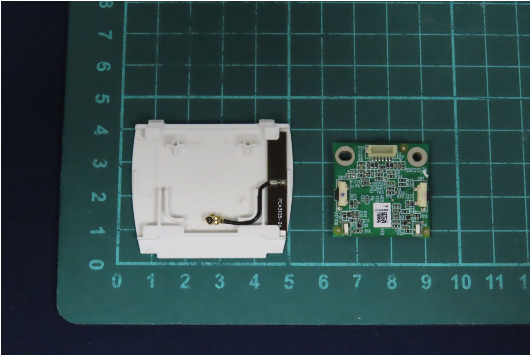
(17) EUT Photo _M/N: MCS1-A
