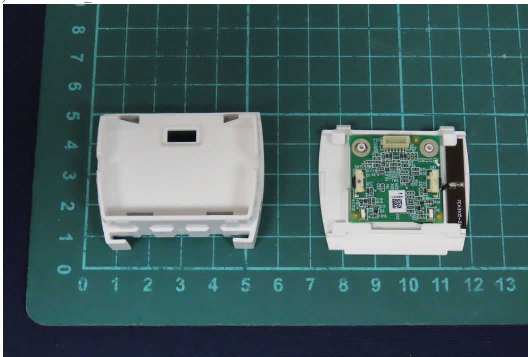
(26) EUT Photo _M/N: MCS1-B
