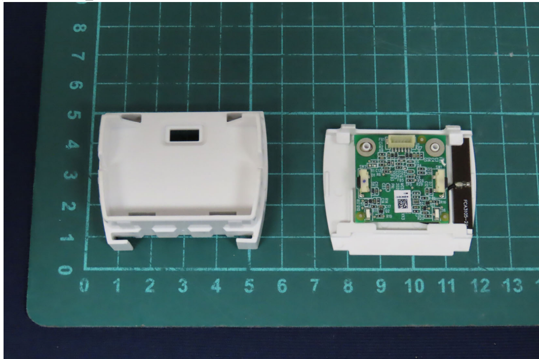
(15) EUT Photo _M/N: MCS1-A
