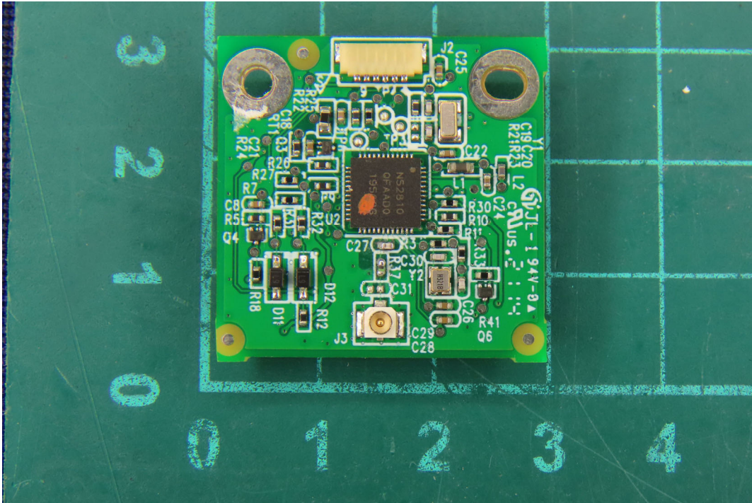
(19) EUT Photo _M/N: MCS1-A
