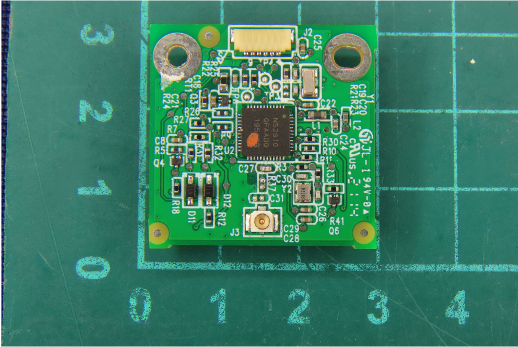
(30) EUT Photo _M/N: MCS1-B
