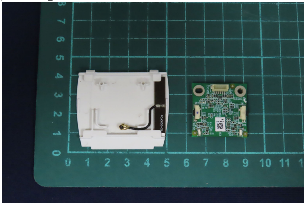
(28) EUT Photo _M/N: MCS1-B
