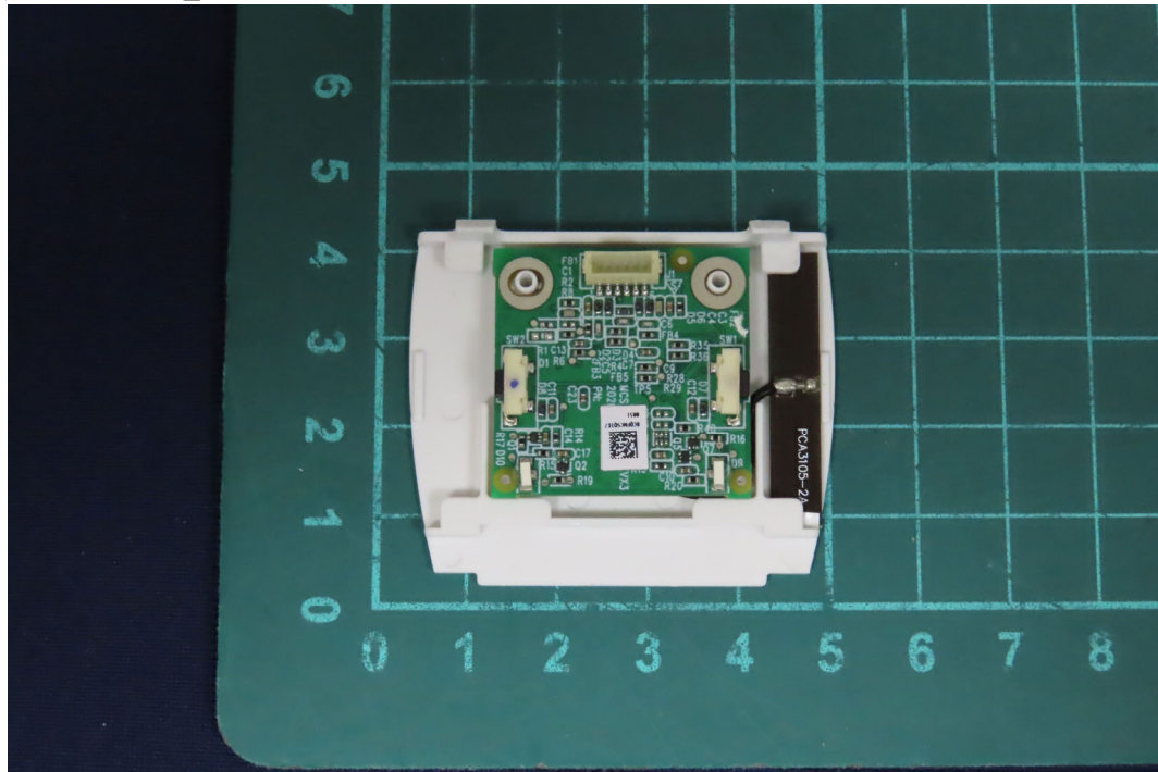
(27) EUT Photo _M/N: MCS1-B
