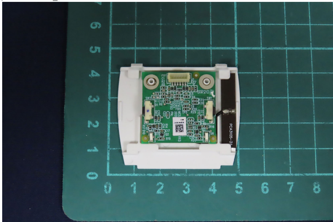
(16) EUT Photo _M/N: MCS1-A
