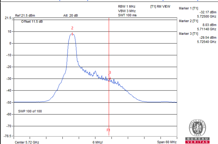
802.11ax (HE20) 26-tone RU / Chain 0 : CH 144 (U-NII-2C)
