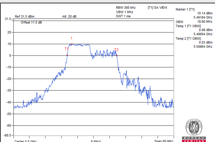
802.11ax (HE20) 106-tone RU / Chain 1 : CH 100
