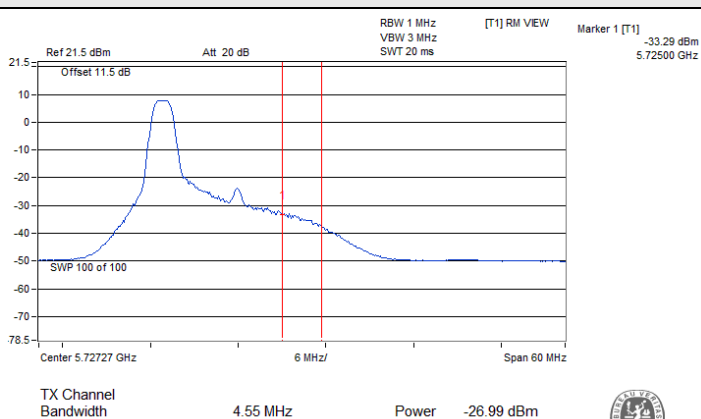
802.11ax (HE20) 26-tone RU / Chain 0 : CH 144 (U-NII-3)
