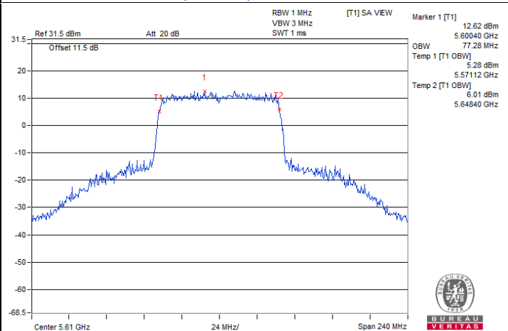
802.11ac (VHT80) / Chain 1 : CH 122
