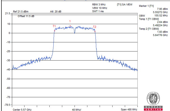
802.11ac (VHT160) / Chain 0 : CH 114
