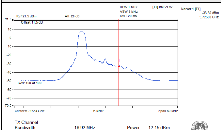
802.11ax (HE20) 26-tone RU / Chain 0 : CH 144 (U-NII-2C)
