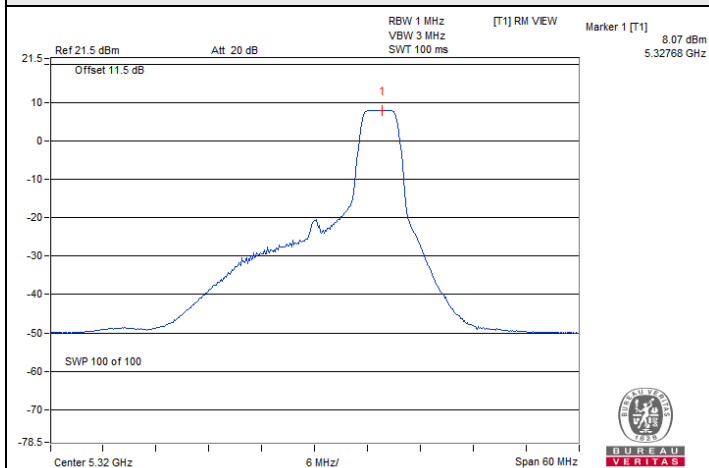
802.11ax (HE20) 52-tone RU / Chain 0 : CH 64
