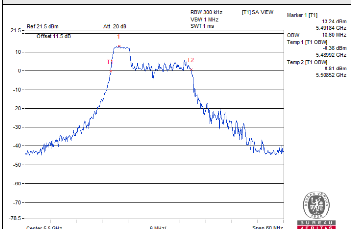
802.11ax (HE20) 52-tone RU / Chain 0 : CH 100
