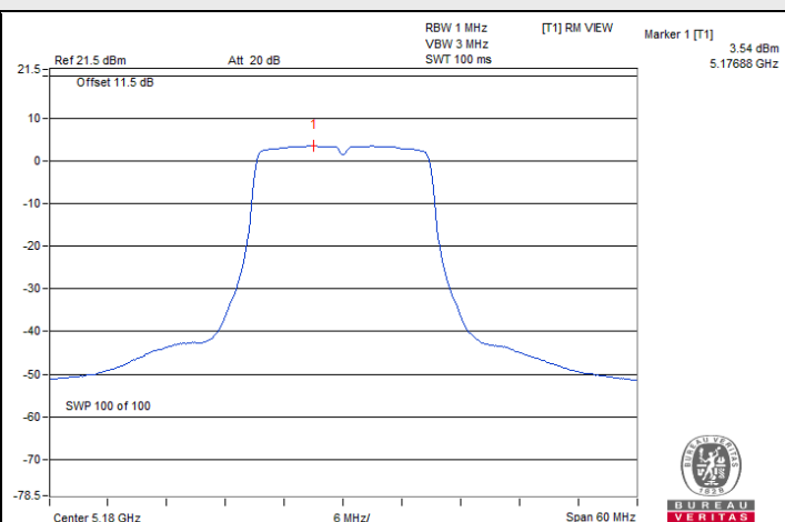
802.11ac (VHT20) / Chain 0 : CH 36
