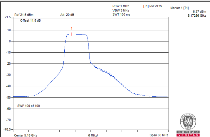
802.11ax (HE20) 106-tone RU / Chain 0 : CH 36
