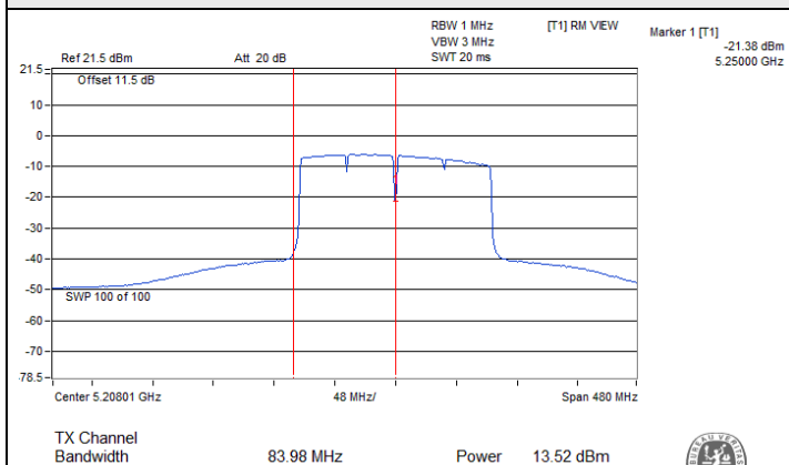
802.11ac (VHT160) / Chain 1 : CH 50 (U-NII-1)
