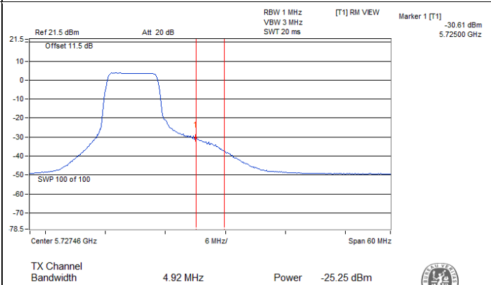
802.11ax (HE20) 106-tone RU / Chain 0 : CH 144 (U-NII-3)
