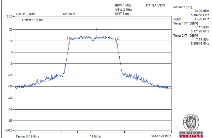
802.11ac (VHT40) / Chain 0 : CH 38
