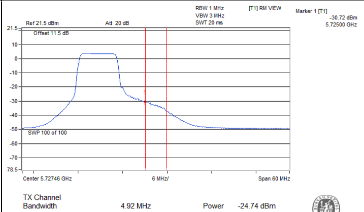
802.11ax (HE20) 52-tone RU / Chain 1 : CH 144 (U-NII-3)
