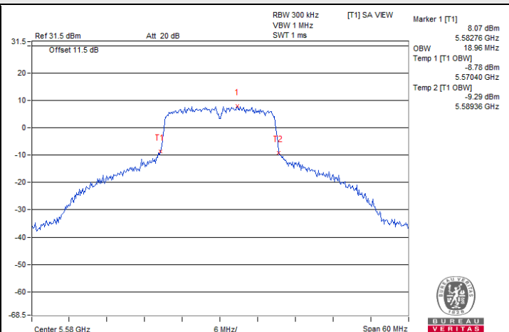
802.11ac (VHT20) / Chain 1 : CH 116
