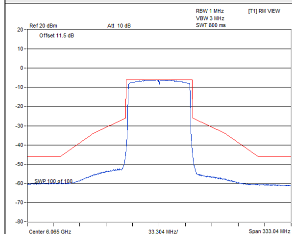
802.11ax (HE80) / Chain 0 : CH 23
