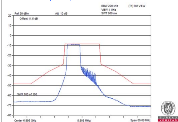
802.11ax (HE20) 106-tone RU / Chain 1 : CH 209
