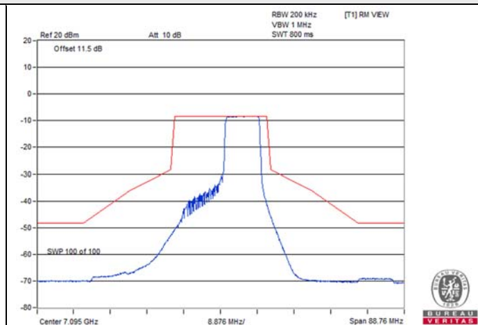
802.11ax (HE20) 106-tone RU / Chain 0 : CH 229
