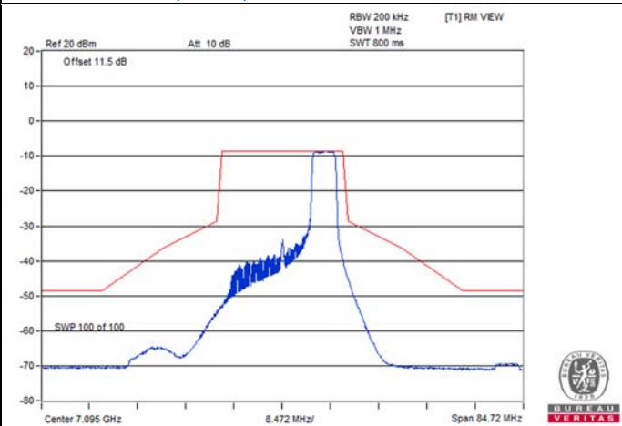
802.11ax (HE20) 52-tone RU / Chain 1 : CH 229
