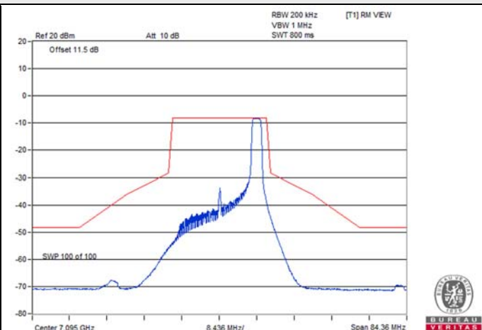
802.11ax (HE20) 26-tone RU / Chain 0 : CH 229
