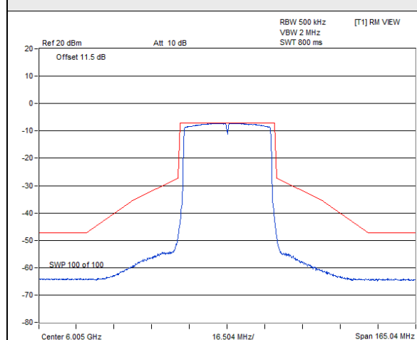
802.11ax (HE40) / Chain 0 : CH 11
