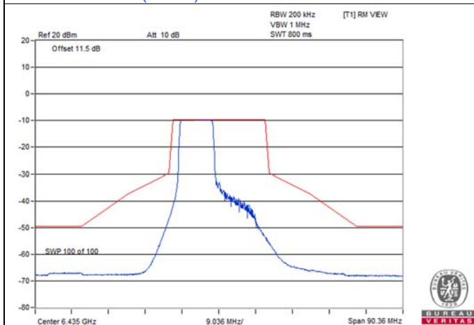
802.11ax (HE20) 106-tone RU / Chain 1 : CH 97
