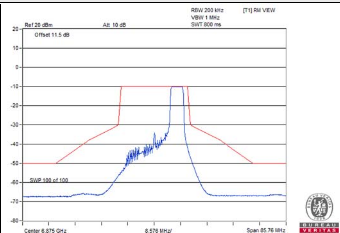
802.11ax (HE20) 52-tone RU / Chain 1 : CH 185
