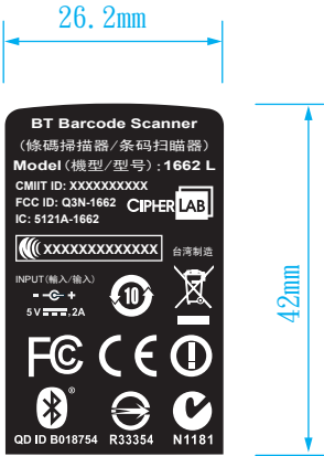
銘版尺寸
