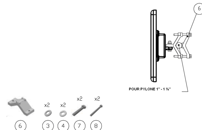
Figure I-4: Montage sur un pylône
