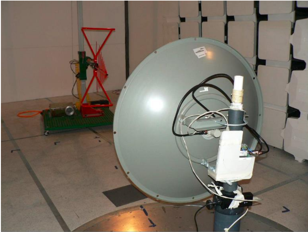
32 dBi Dish RW-9732-4958 Dig Em 30-1000 Front
