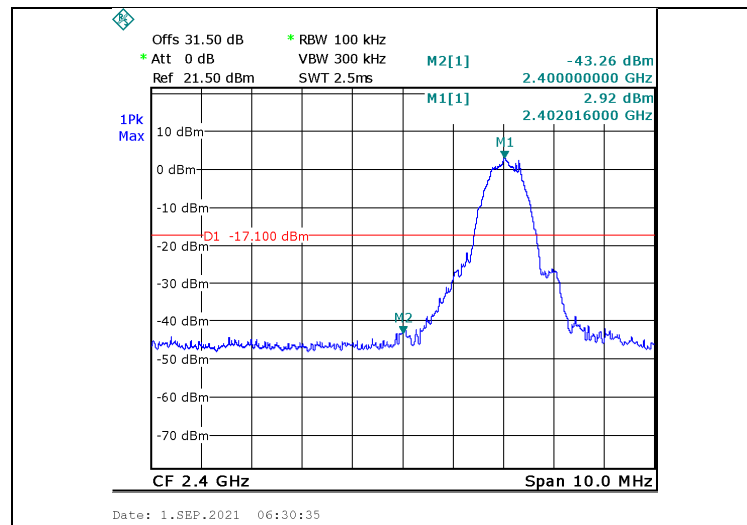
Figure 23. 2402.0 MHz, BLE
