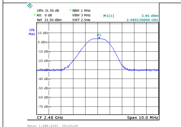
Figure 20. 2480.0 MHz, BLE
