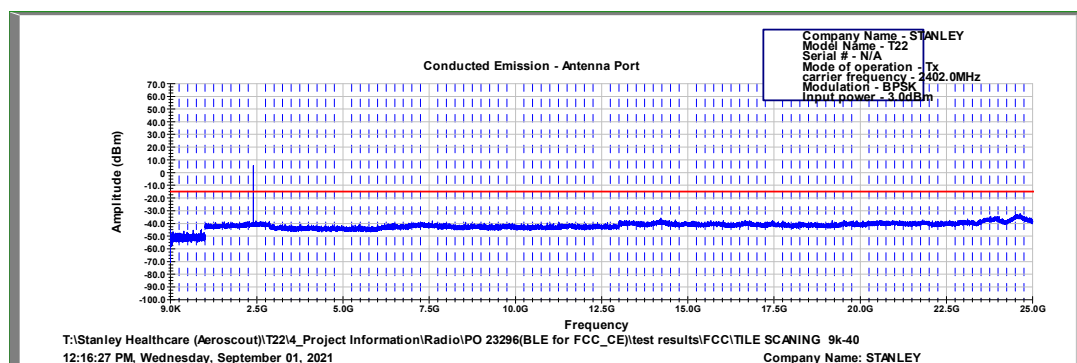
Figure 36 2402.0 MHz, BLE
