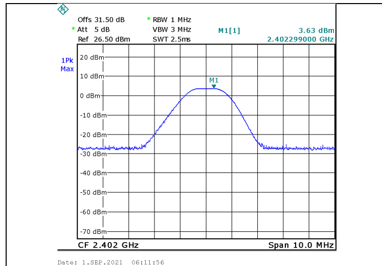
Figure 18. 2402.0 MHz, BLE
