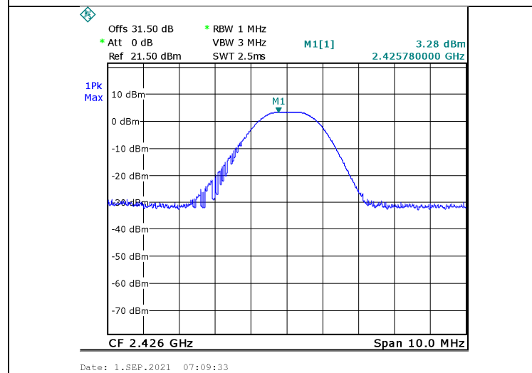
Figure 19. 2426.0 MHz, BLE
