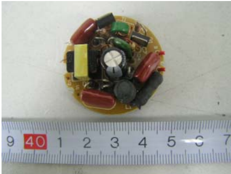
MAE-SP-7WL (D): EUT-PCB Bottom View
