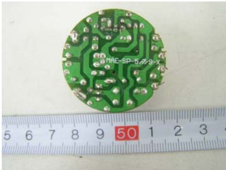
MAE-SP-9WL (D): EUT-PB Bottom View
