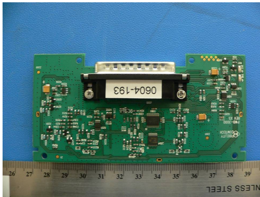
EUT - T/R Module Component side
