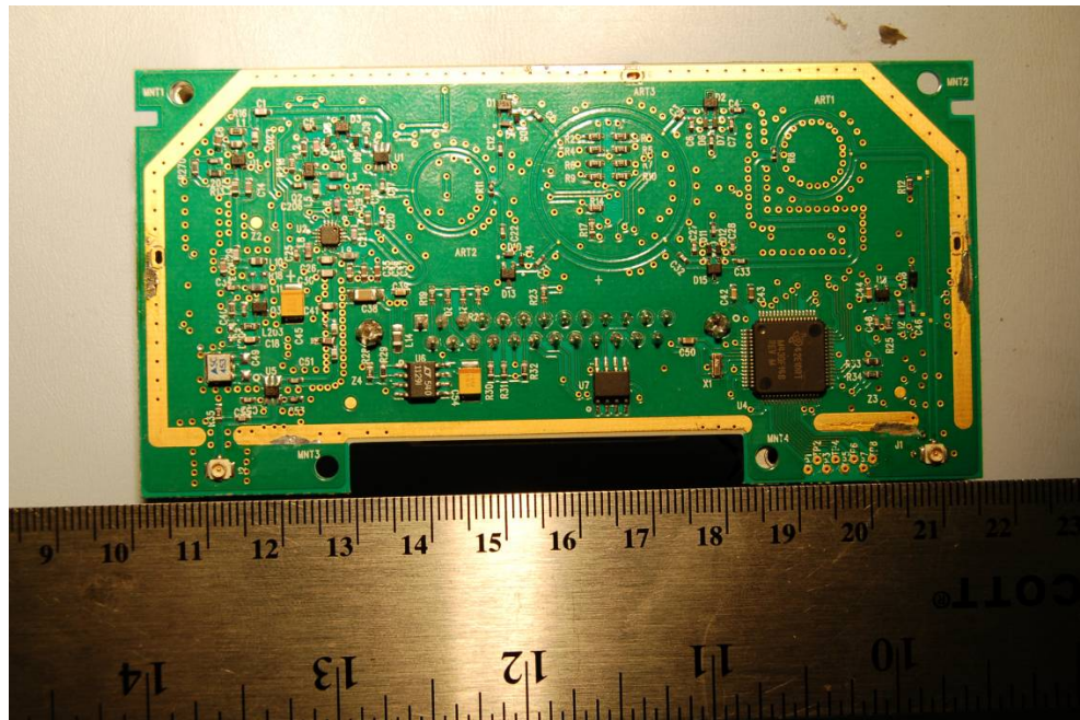
EUT - T/R Module Solder side
