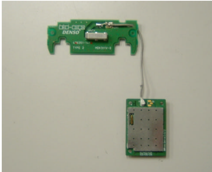
Module + Antenna
