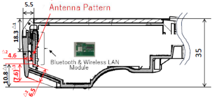
Bluetooth & Wireless LAN Module
