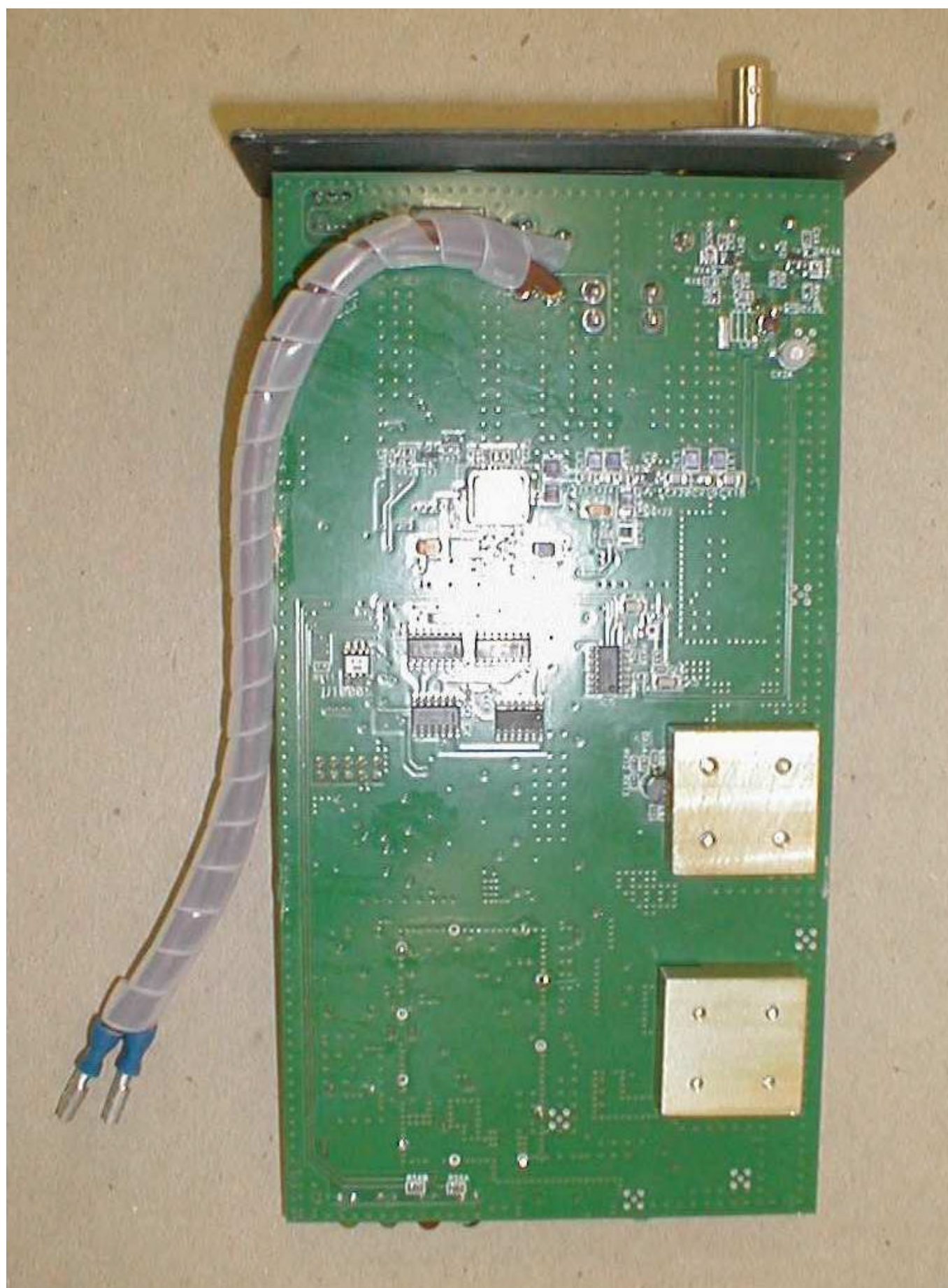
PCB Bottom
