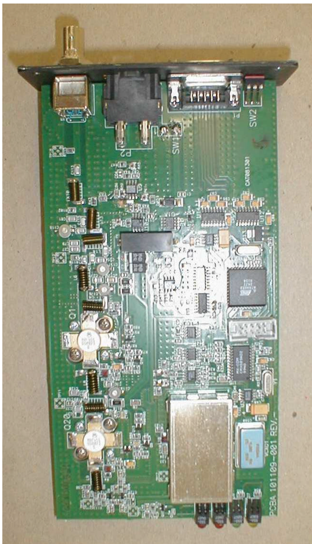
PCB Top
