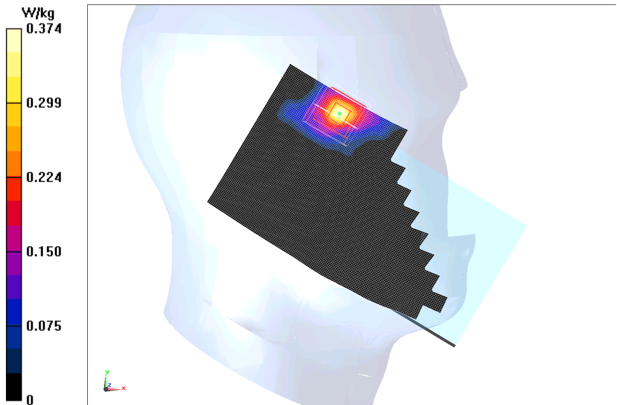
Fig.24 5GHz CH48
