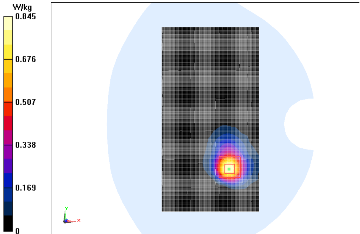
Fig.25 5GHz CH52
