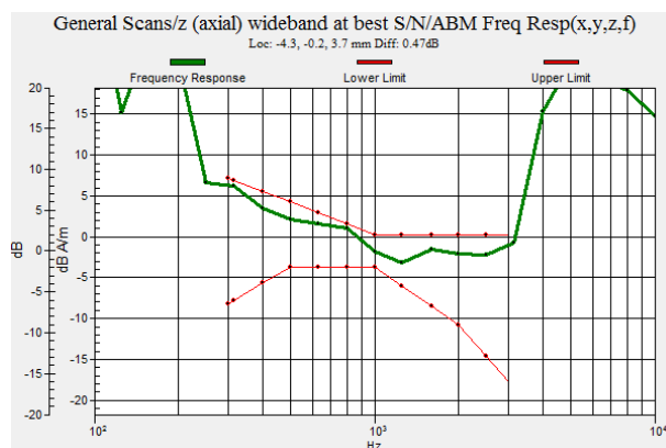
Fig 9.6 GSM1900 Ch810
