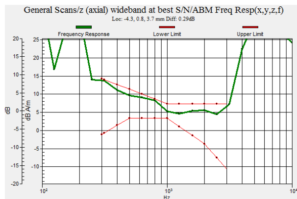
Fig 9.2 GSM850 Ch189
