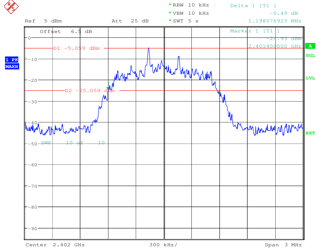
Plot 4 Pi/4 DQPSK
