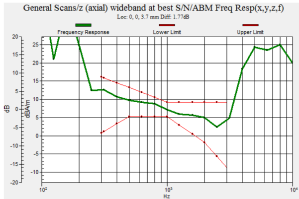
Fig 7.1 GSM850 Ch189
