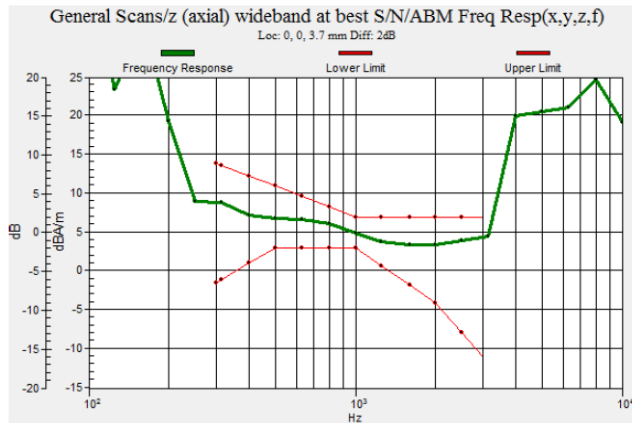
Fig 7.3 WCDMA Band II Ch9400
