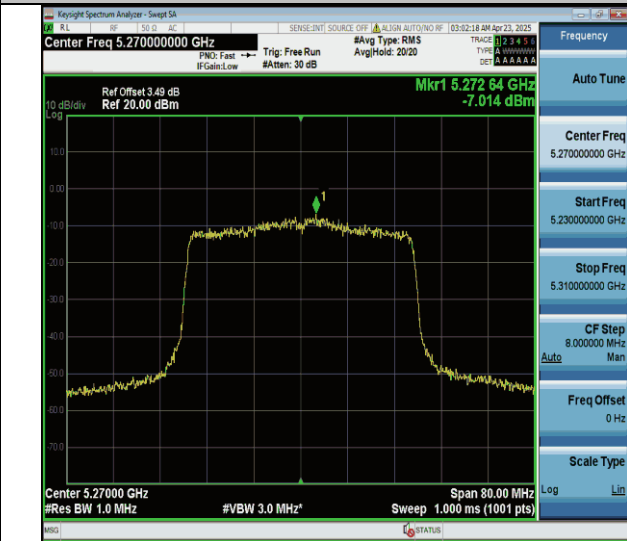
11ax40MIMO-Ant7-5270-PASS
