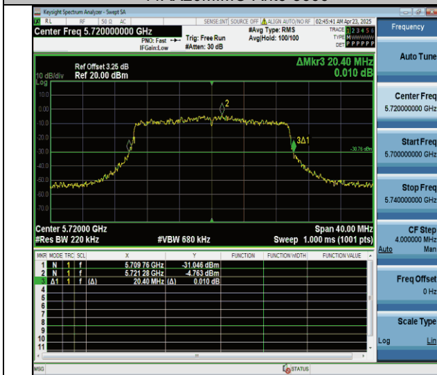
11ax20MIMO-Ant6-5720
