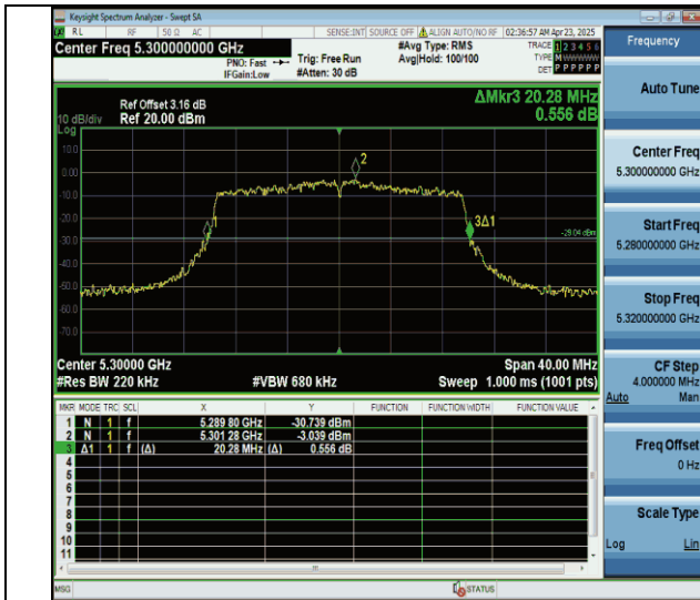
11ax20MIMO-Ant6-5300
