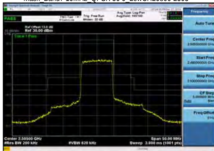
Mask Band7 10MHz QPSK 50 0 LowCH20800-2505
