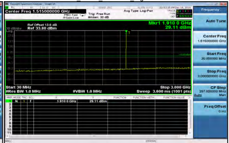
30MHz-3GHz EDGE 1900MHz HighCH810-1909.8
