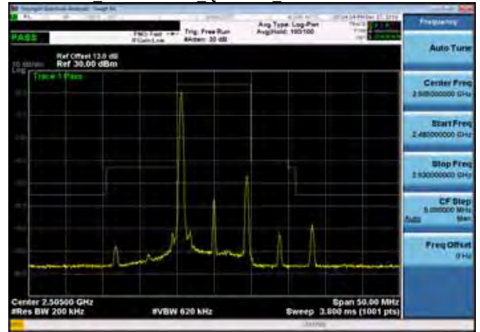
Mask Band7 10MHz QPSK 1 0 LowCH20800-2505
