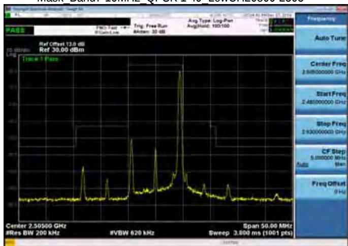
Mask Band7 10MHz QPSK 1 49 LowCH20800-2505
