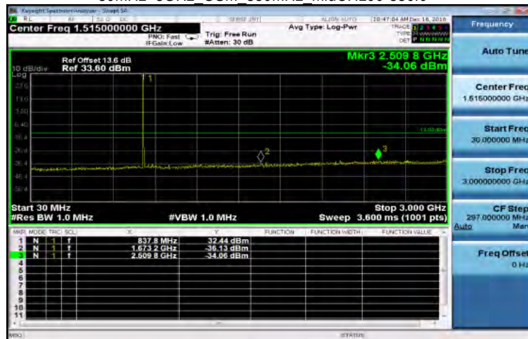
30MHz~3GHz GSM 850MHz MidCH190-836.6
