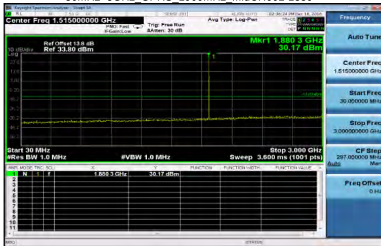
30MHz-3GHz GPRS 1900MHz MidCH661-1880
