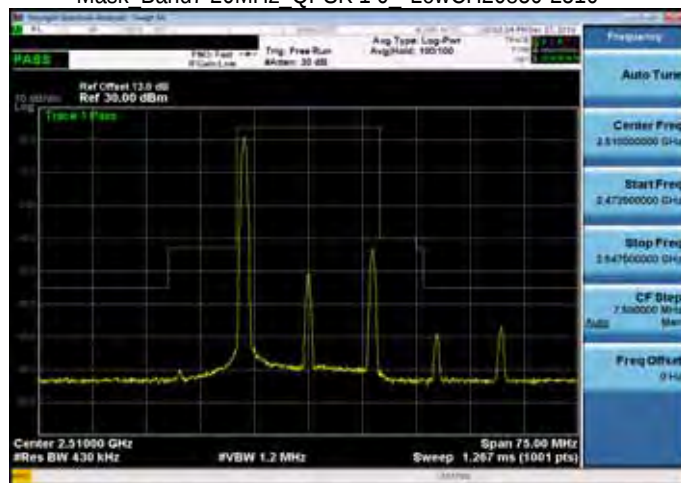
Mask Band7 20MHz_QPSK 1 0_LowCH20850-2510
