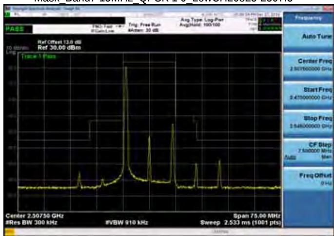
Mask Band7 15MHz_QPSK 1 0_LowCH20825-2507.5
