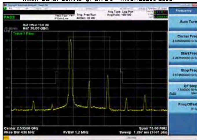
Mask Band7 20MHz_QPSK 1 0_MidCH21100-2535
