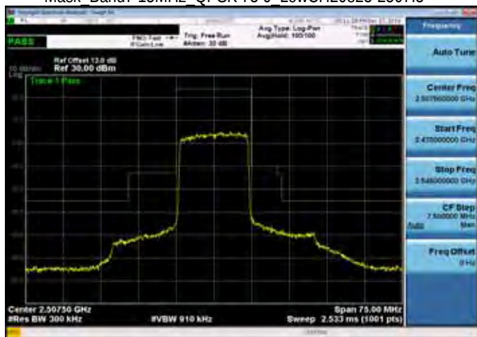
Mask Band7 15MHz_QPSK 75 0_LowCH20825-2507.5
