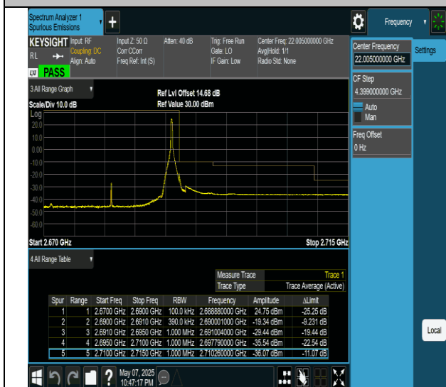
Band41-20MHz-QPSK-41490-1RB#99-PASS
