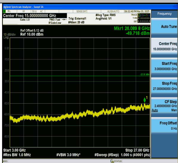
Band41-20MHz-QPSK-41490-1RB#0-3000~27000-PASS
