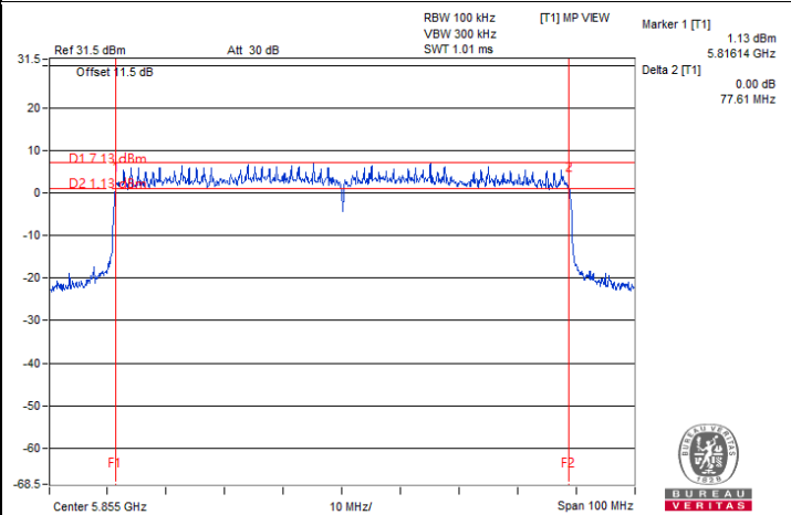
802.11be (EHT80) Beamforming / Chain 2 : CH 171
