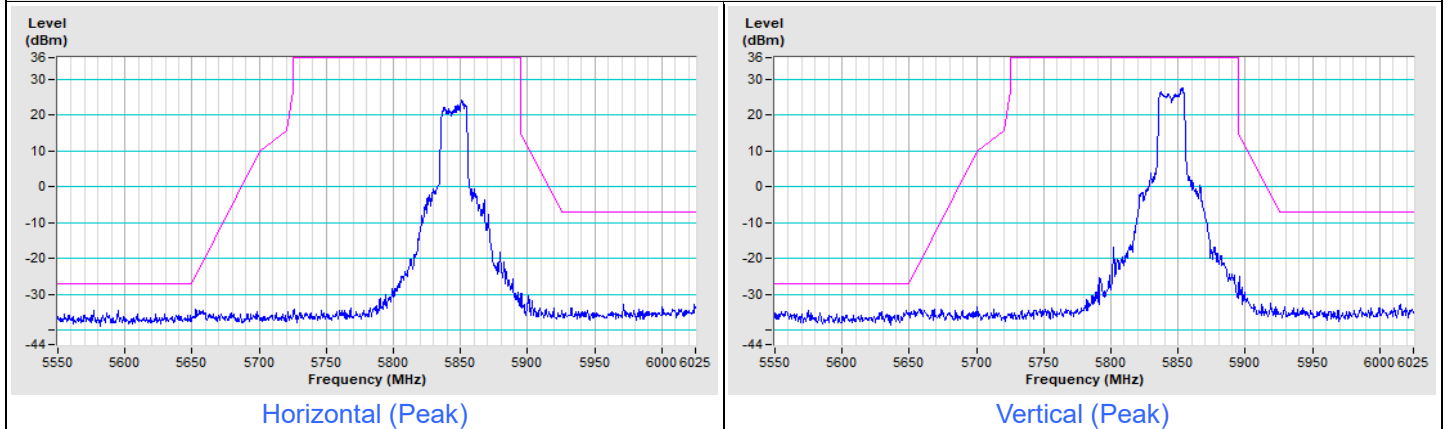
802.11be (EHT20) Beamforming Channel 169
