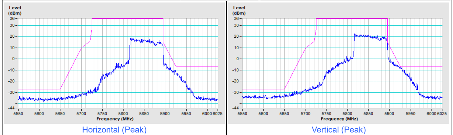
802.11be (EHT80) Beamforming Channel 171
