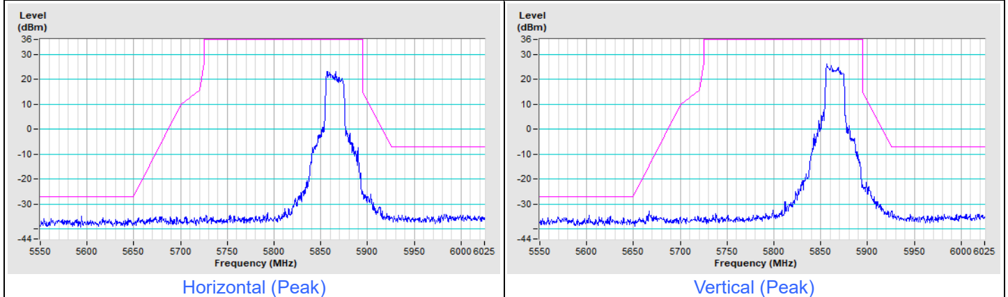
802.11be (EHT20) Beamforming Channel 173
