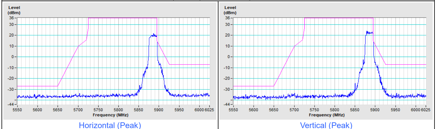
802.11be (EHT20) Beamforming Channel 177
