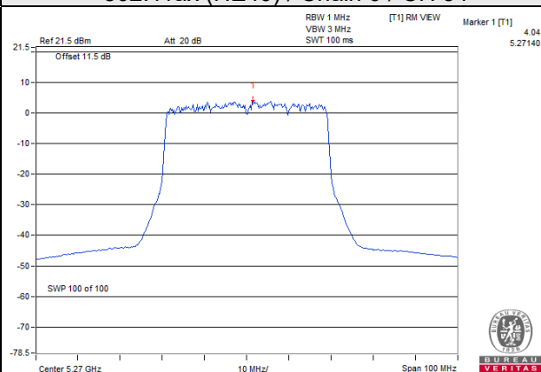
802.11ax (HE40) / Chain 0 / CH 54
