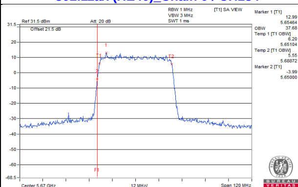
802.11ax (HE40)_Chain 2 / CH134
