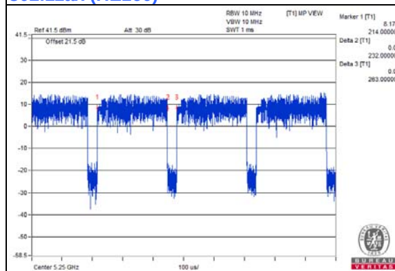
802.11ax (HE160)
