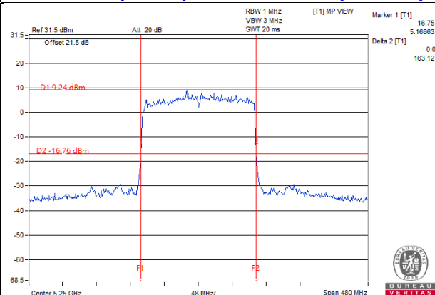
802.11ax (HE160)_Chain 3 / CH50 (U-NII-2A)
