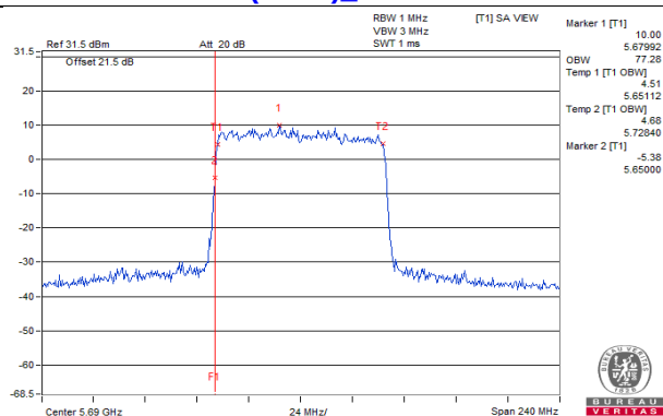
802.11ax (HE80)_Chain 2 / CH138
