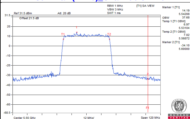
802.11ax (HE40)_Chain 2 / CH110
