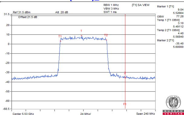
802.11ax (HE80)_Chain 2 / CH106
