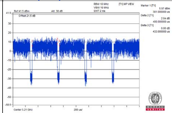
802.11ax (HE80)
