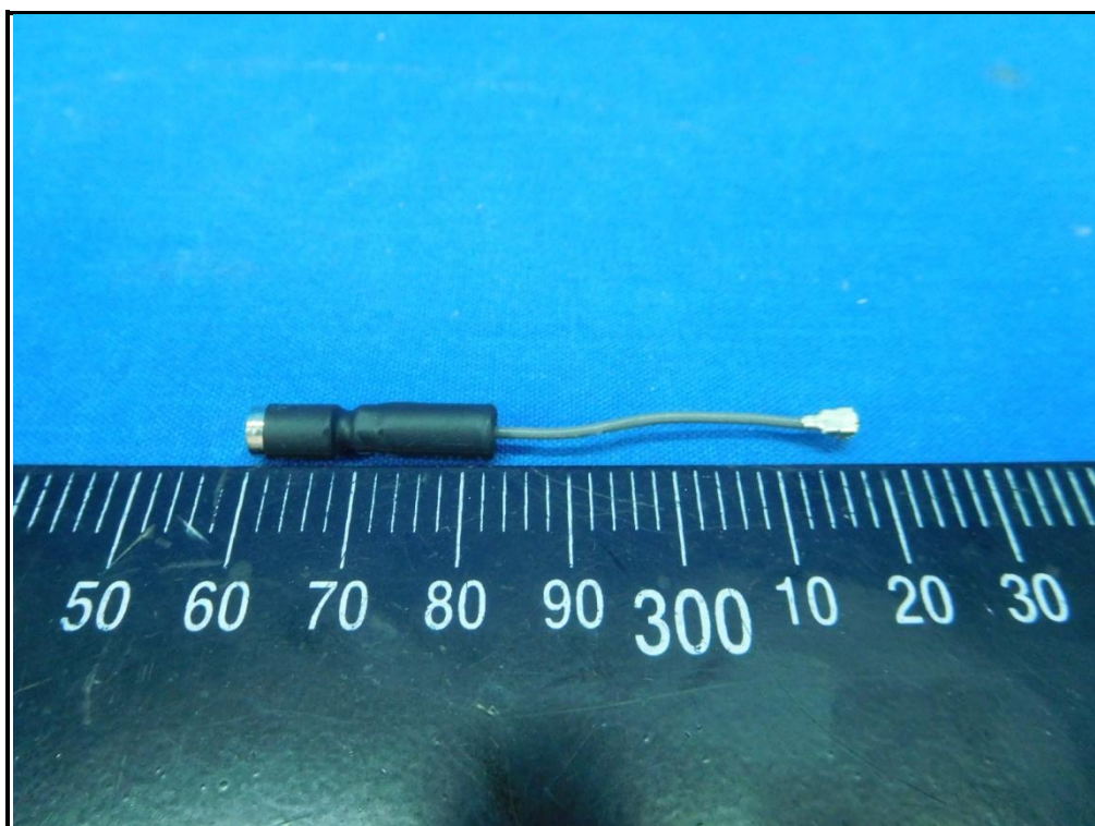
Antenna: 5GHz_Chain 1
