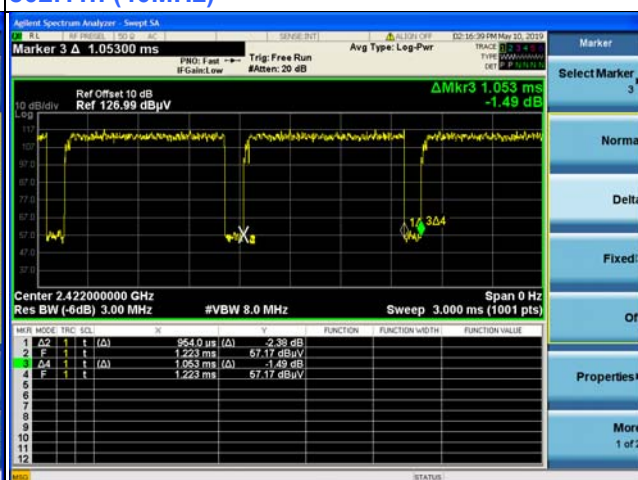
802.11n (40MHz)
