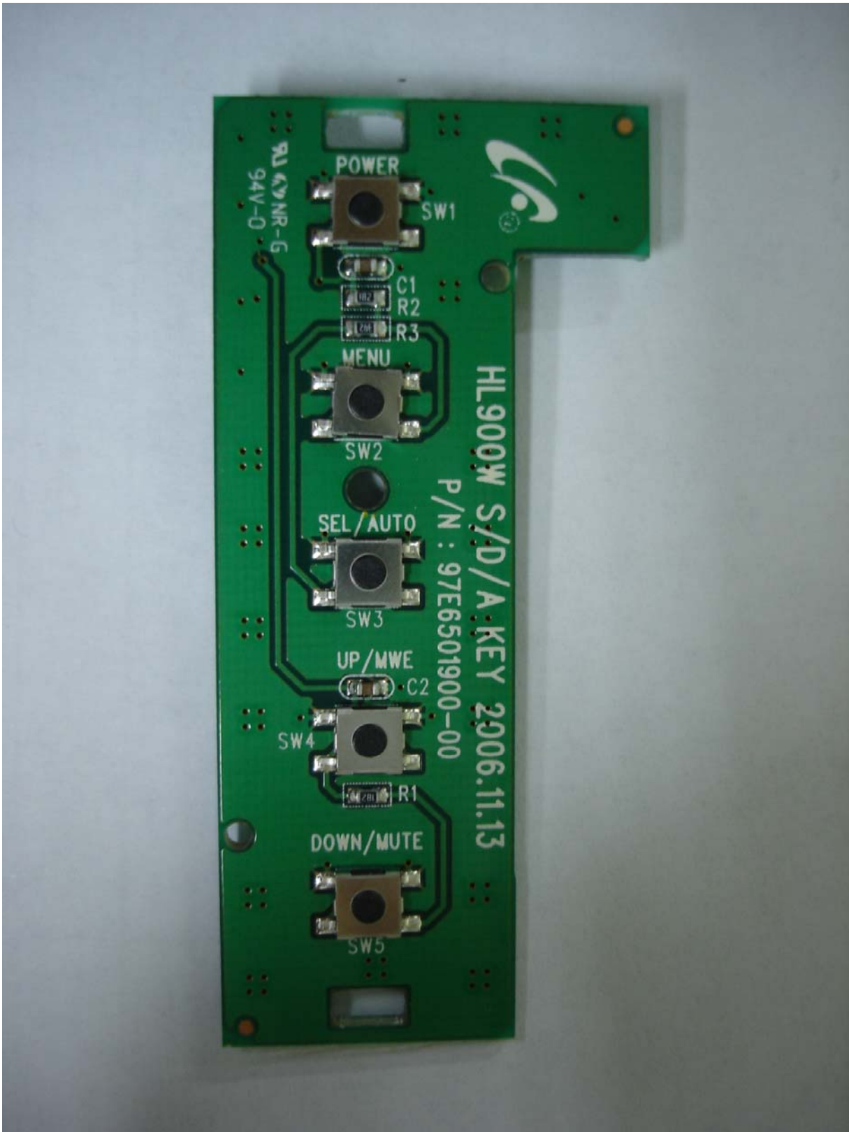
<Key Front>
