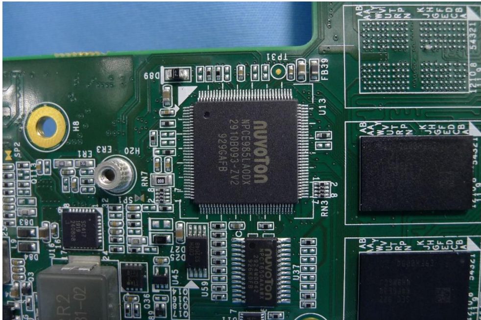
(36) EUT Photo
