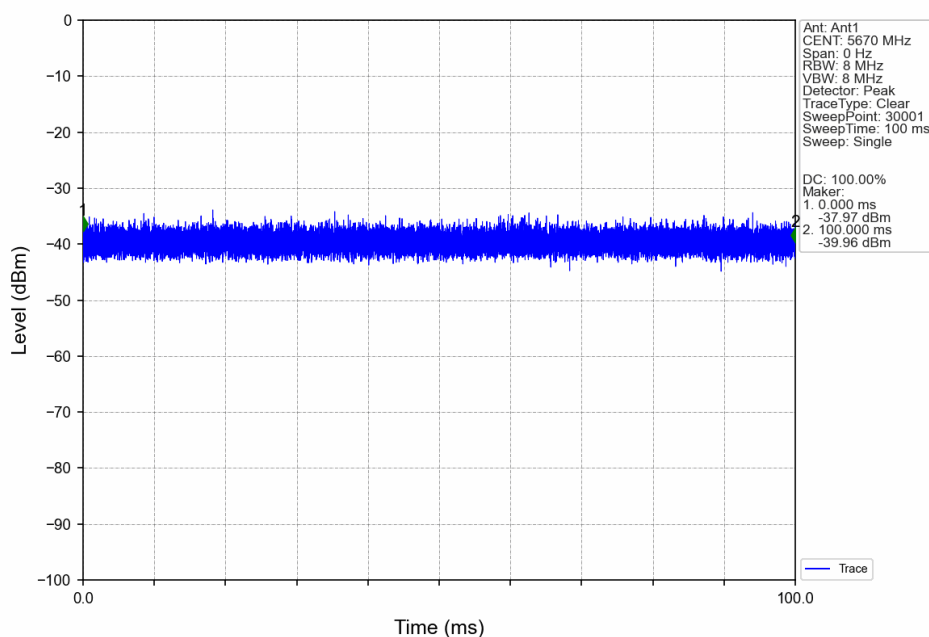
802.11ax(HEW40)_HCH_5670MHz_RU484_Left_Ant1_NTNV
