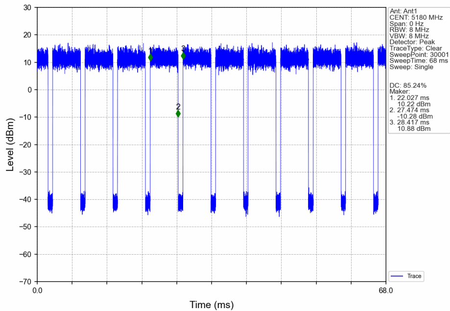
802.11ax(HEW20)_LCH_5180MHz_RU242_Left_Ant1_NTNV
