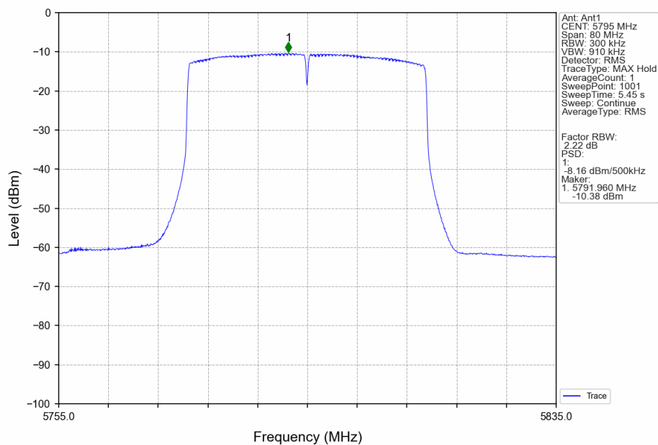
802.11ax(HEW40)_HCH_5795MHz_RU26_Left_Ant1_NTNV
