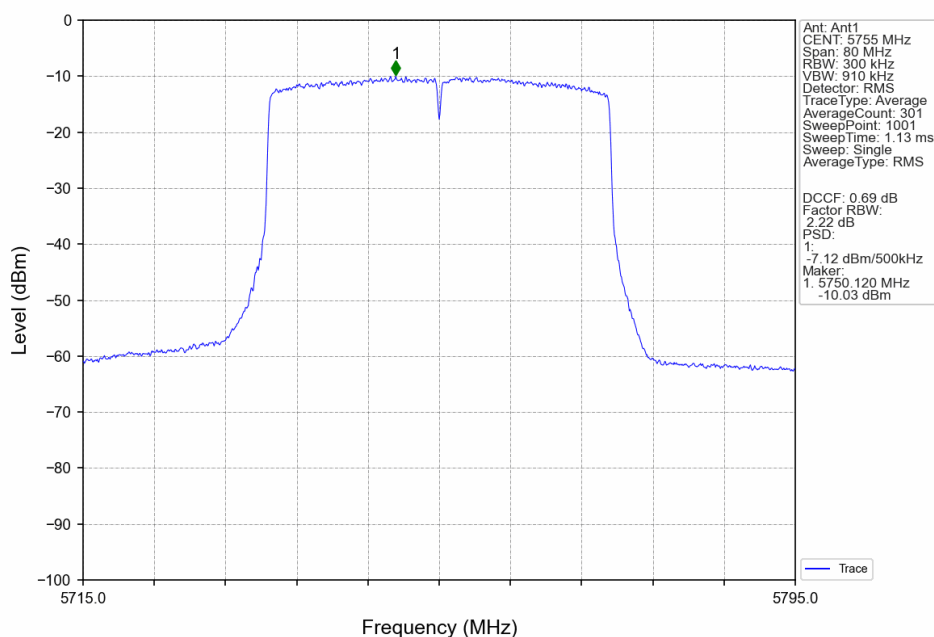
802.11ax(HEW40)_LCH_5755MHz_RU26_Left_Ant1_NTNV
