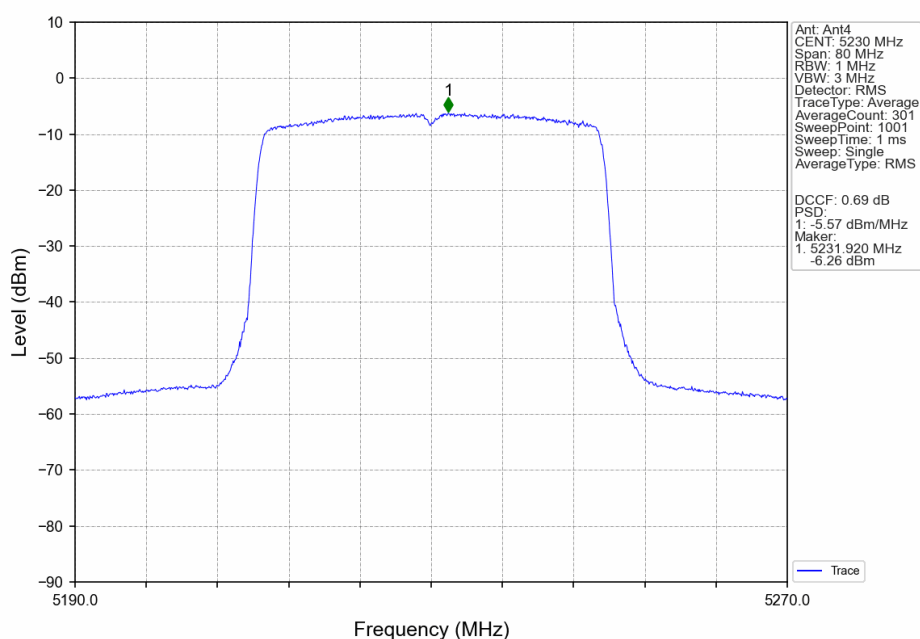
802.11ax(HEW40)_HCH_5230MHz_RU26_Left_Ant4_NTNV
