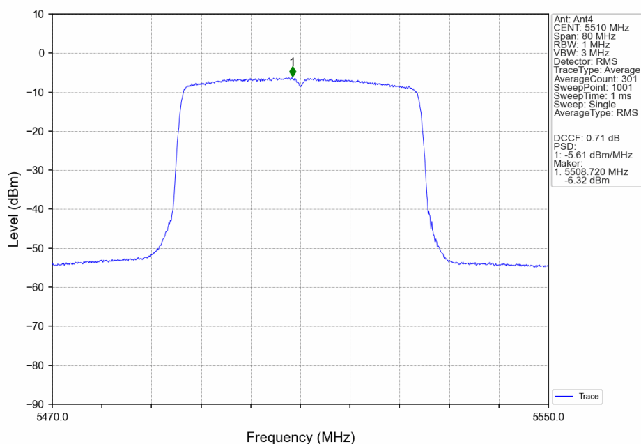
802.11ax(HEW40)_LCH_5510MHz_RU26_Left_Ant4_NTNV
