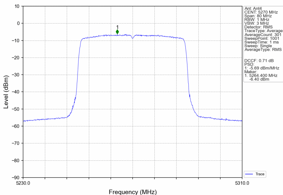
802.11ax(HEW40)_LCH_5270MHz_RU26_Right_Ant4_NTNV
