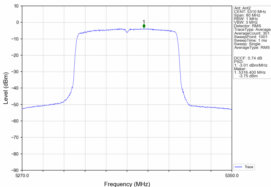
802.11ax(HEW40)_HCH_5310MHz_RU26_Left_Ant2_NTNV
