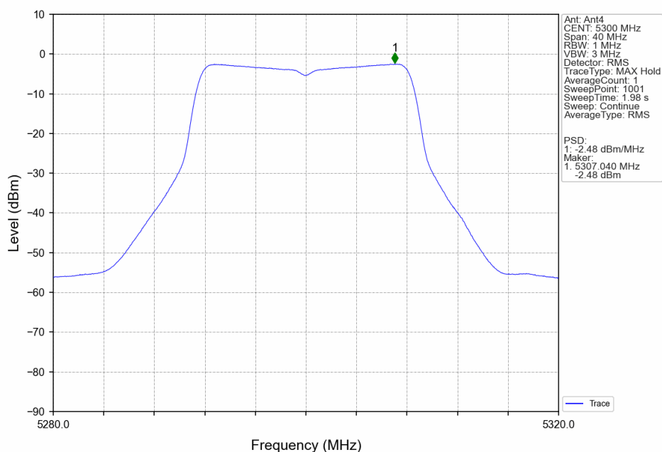
802.11a_MCH_5300MHz_Ant4_NTNV
