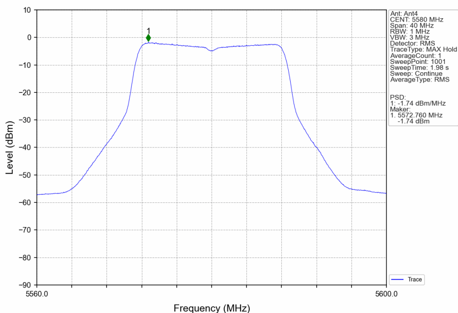
802.11a_MCH_5580MHz_Ant4_NTNV
