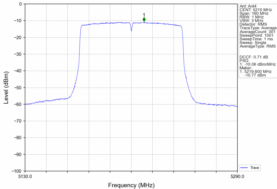
802.11ac(VHT80)_MCH_5210MHz_MIMO_NTNV
