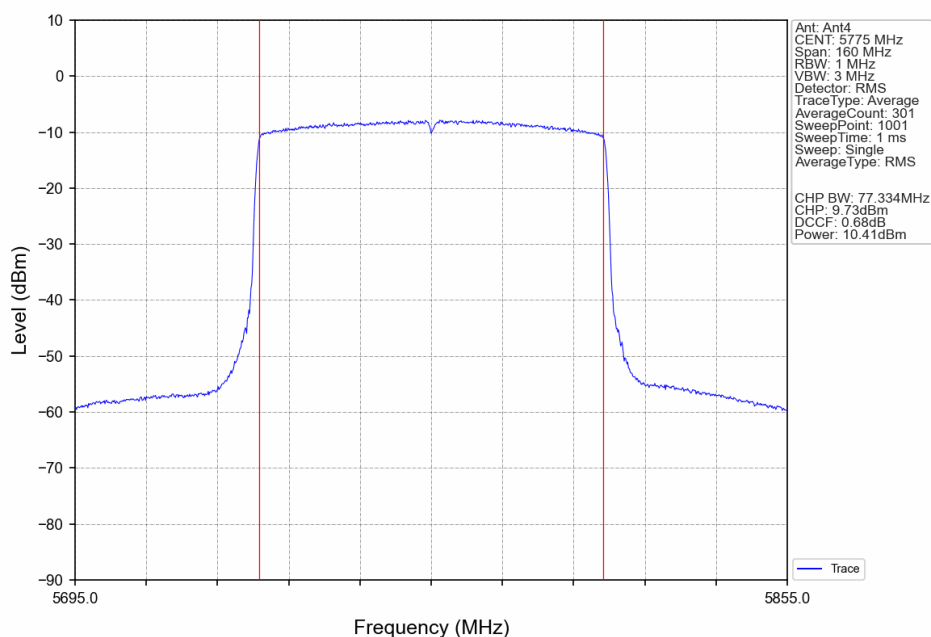
802.11ax(HEW80)_MCH_5775MHz_RU996_Left_Ant4_NTNV
