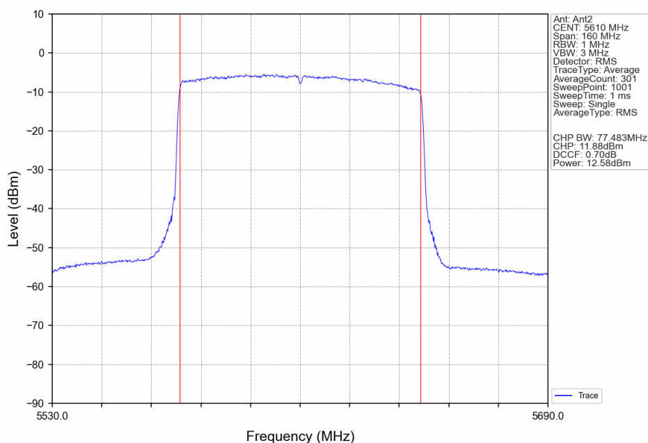
802.11ax(HEW80)_HCH_5610MHz_RU996_Left_Ant2_NTNV
