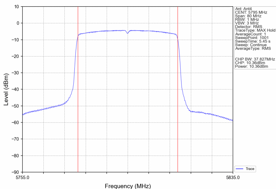
802.11ax(HEW40)_HCH_5795MHz_RU484_Left_Ant4_NTNV
