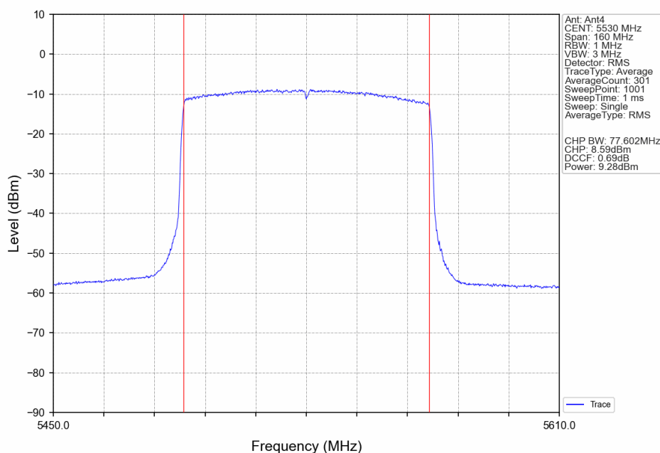
802.11ax(HEW80)_LCH_5530MHz_RU996_Left_Ant4_NTNV
