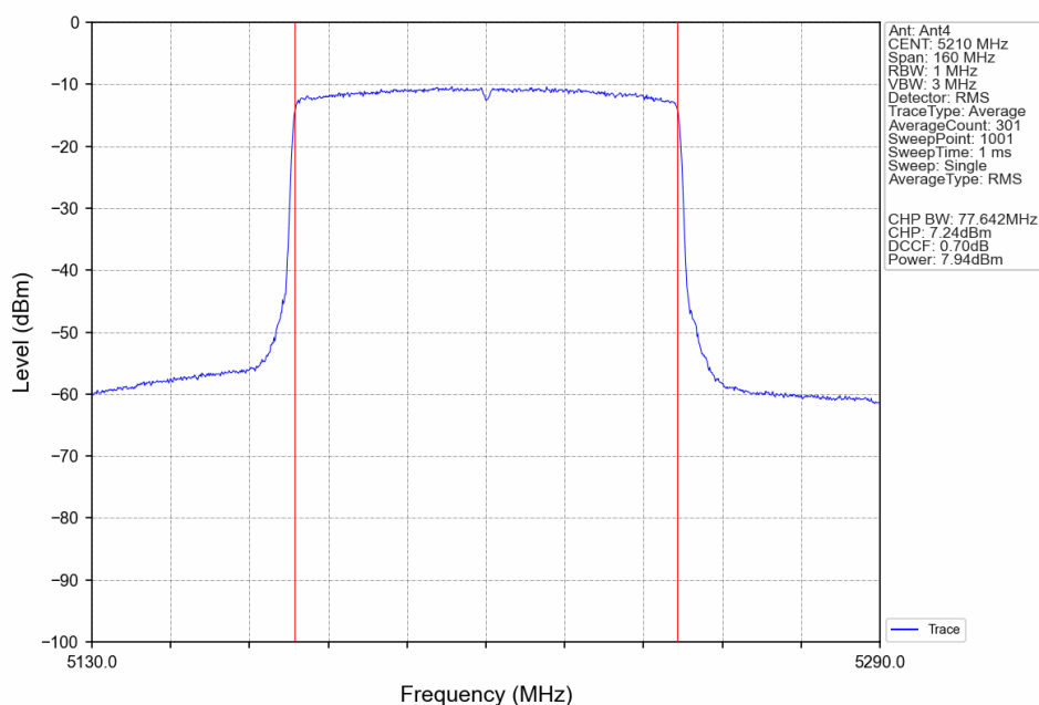
802.11ax(HEW80)_MCH_5210MHz_RU996_Left_Ant4_NTNV
