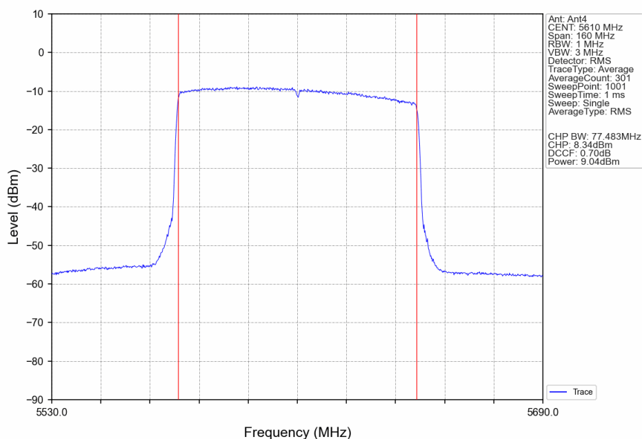
802.11ax(HEW80)_HCH_5610MHz_RU26_Right_Ant4_NTNV
