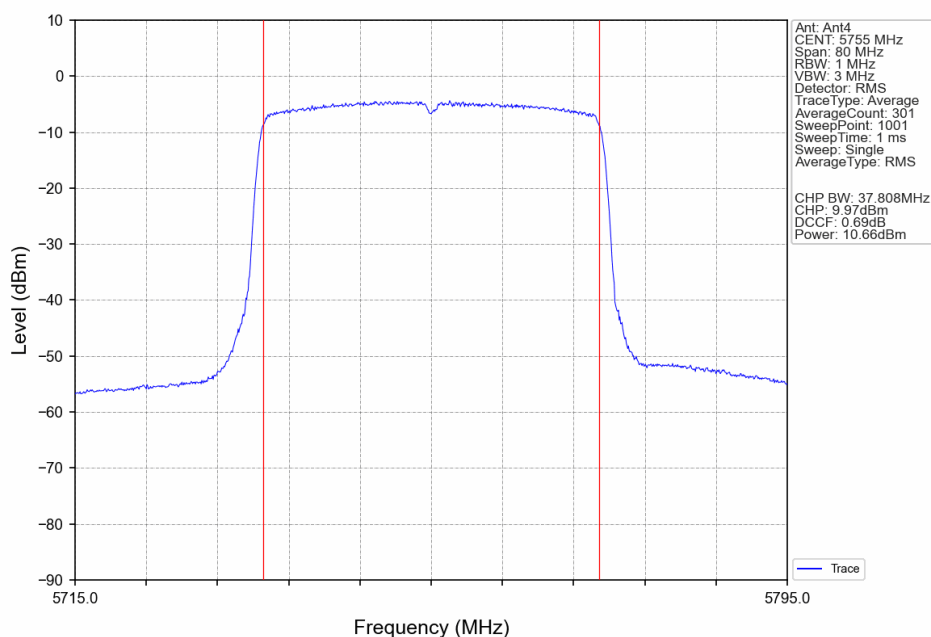
802.11ax(HEW40)_LCH_5755MHz_RU26_Left_Ant4_NTNV
