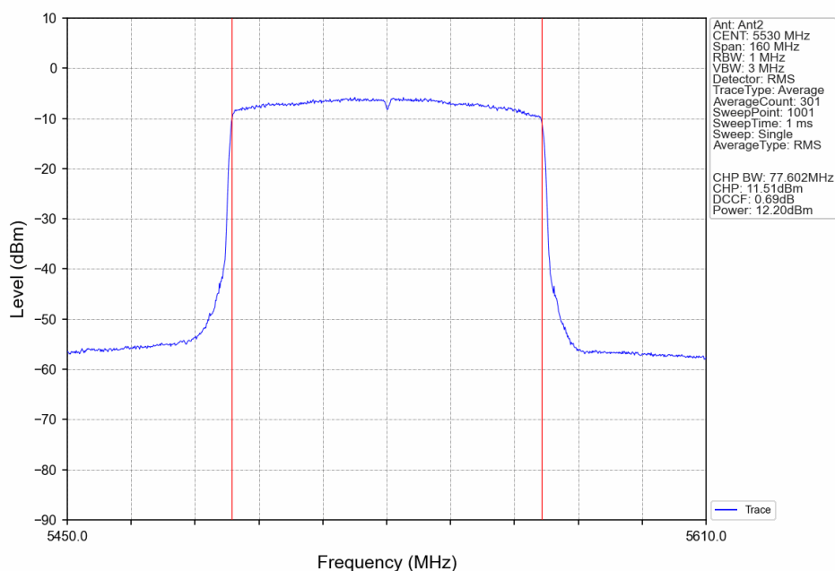
802.11ax(HEW80)_LCH_5530MHz_RU26_Right_Ant2_NTNV
