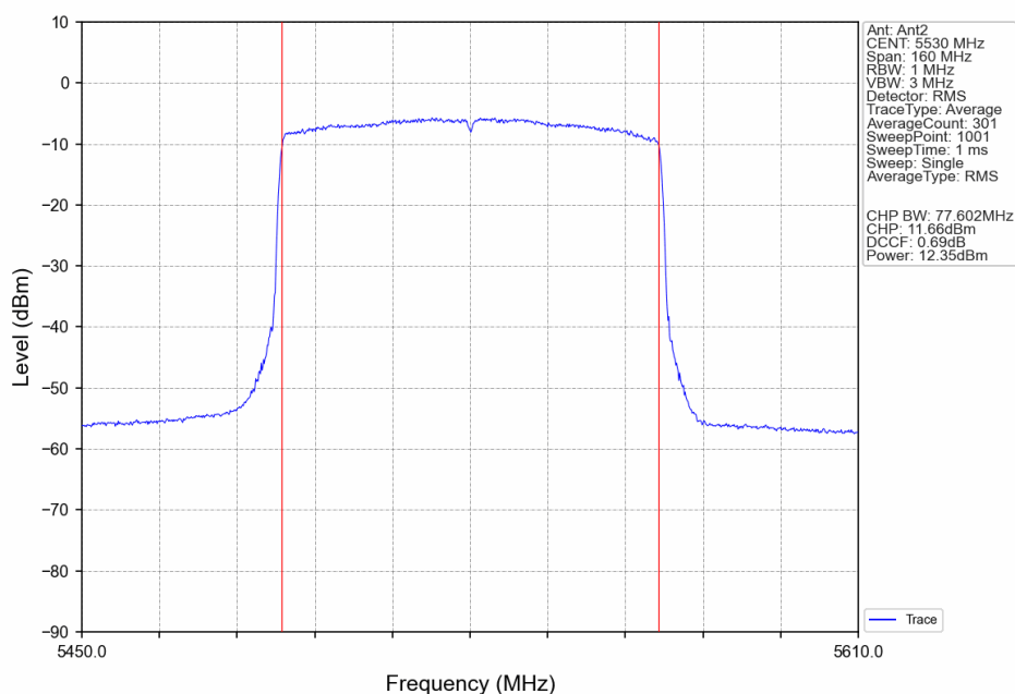
802.11ax(HEW80)_LCH_5530MHz_RU996_Left_Ant2_NTNV
