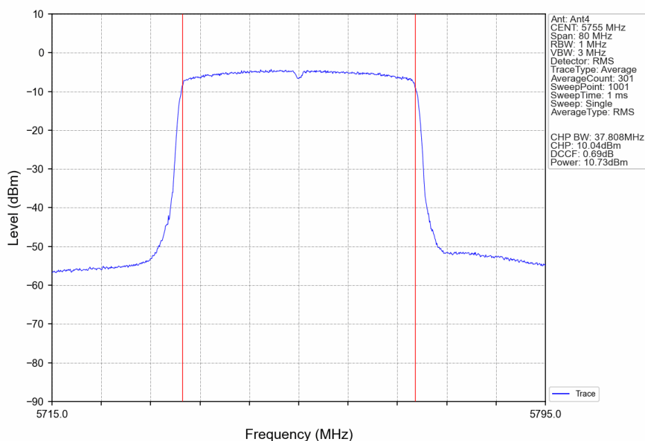
802.11ax(HEW40)_LCH_5755MHz_RU484_Left_Ant4_NTNV
