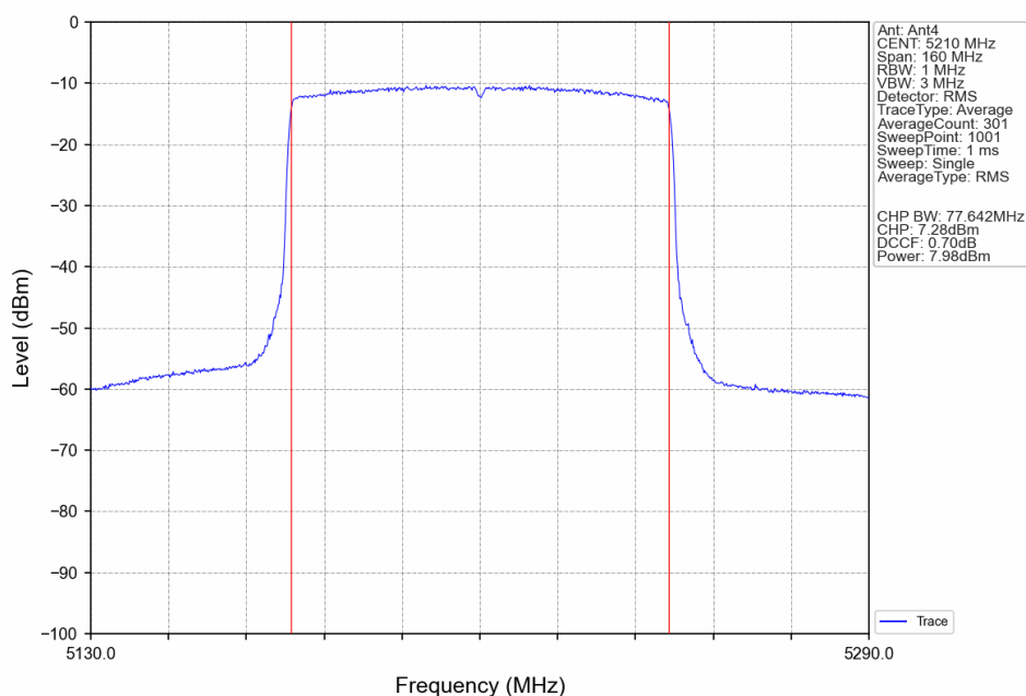
802.11ax(HEW80)_MCH_5210MHz_RU26_Right_Ant4_NTNV
