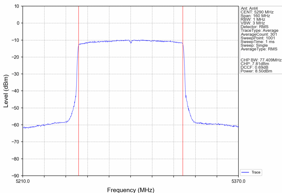
802.11ax(HEW80)_MCH_5290MHz_RU996_Left_Ant4_NTNV
