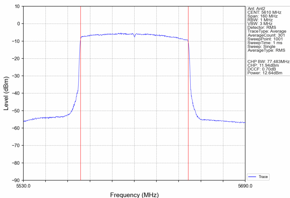
802.11ax(HEW80)_HCH_5610MHz_RU26_Right_Ant2_NTNV
