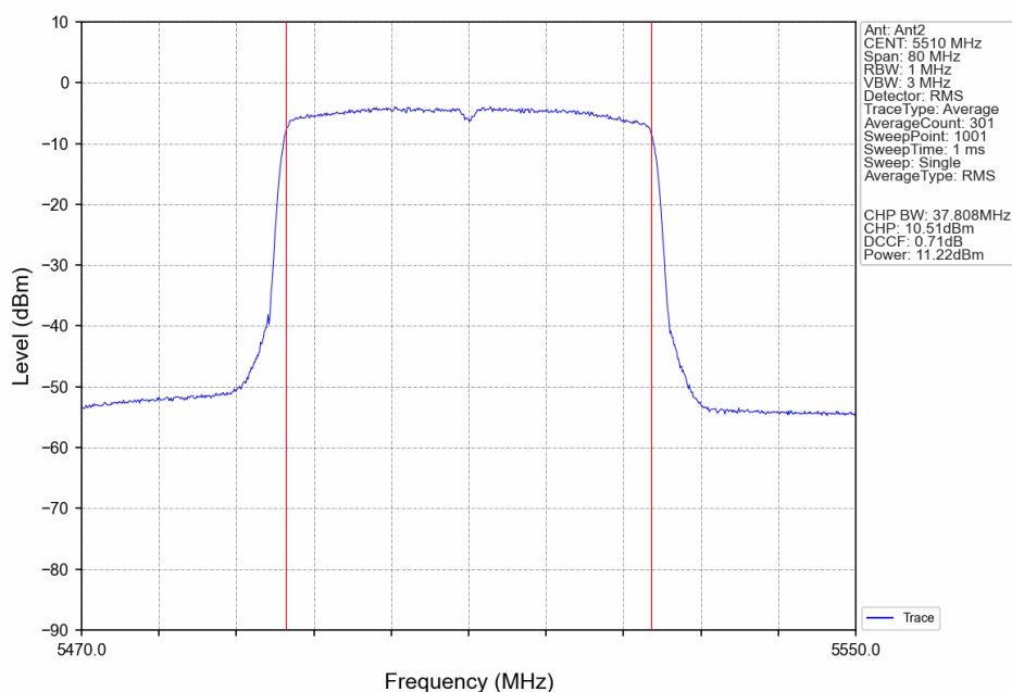
802.11ax(HEW40)_LCH_5510MHz_RU484_Left_Ant2_NTNV
