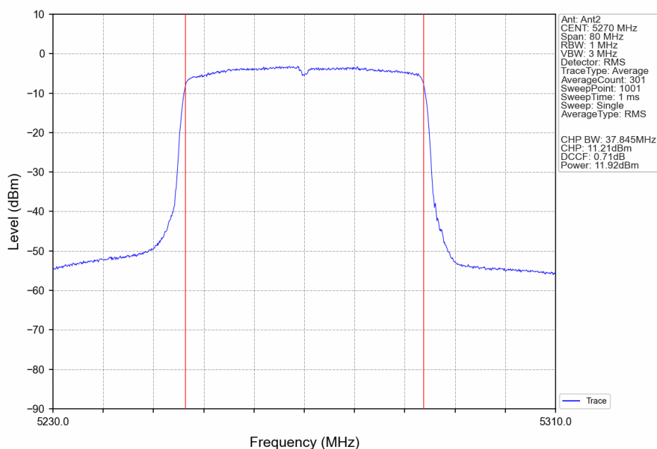
802.11ax(HEW40)_LCH_5270MHz_RU484_Left_Ant2_NTNV
