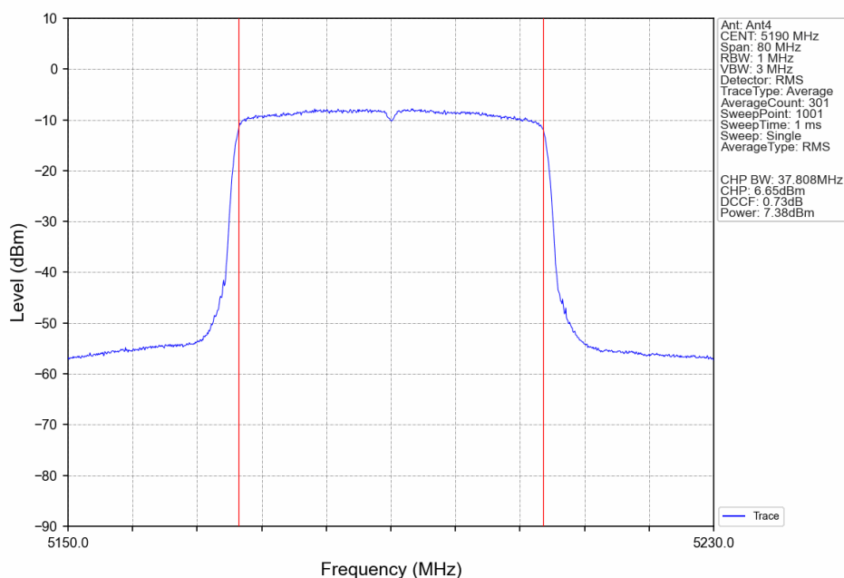
802.11ax(HEW40)_LCH_5190MHz_RU26_Left_Ant4_NTNV
