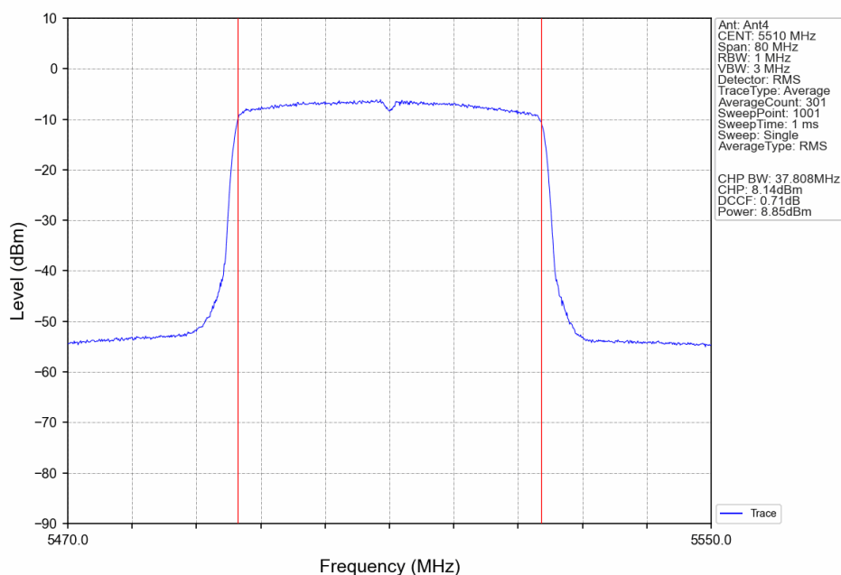
802.11ax(HEW40)_LCH_5510MHz_RU484_Left_Ant4_NTNV
