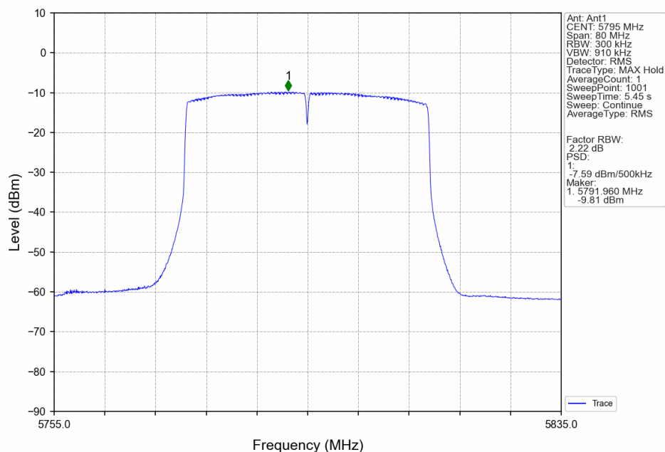
802.11ax(HEW40)_HCH_5795MHz_RU26_Left_Ant1_NTNV
