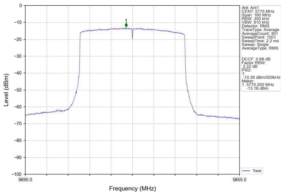
802.11ax(HEW80)_MCH_5775MHz_RU26_Left_Ant1_NTNV
