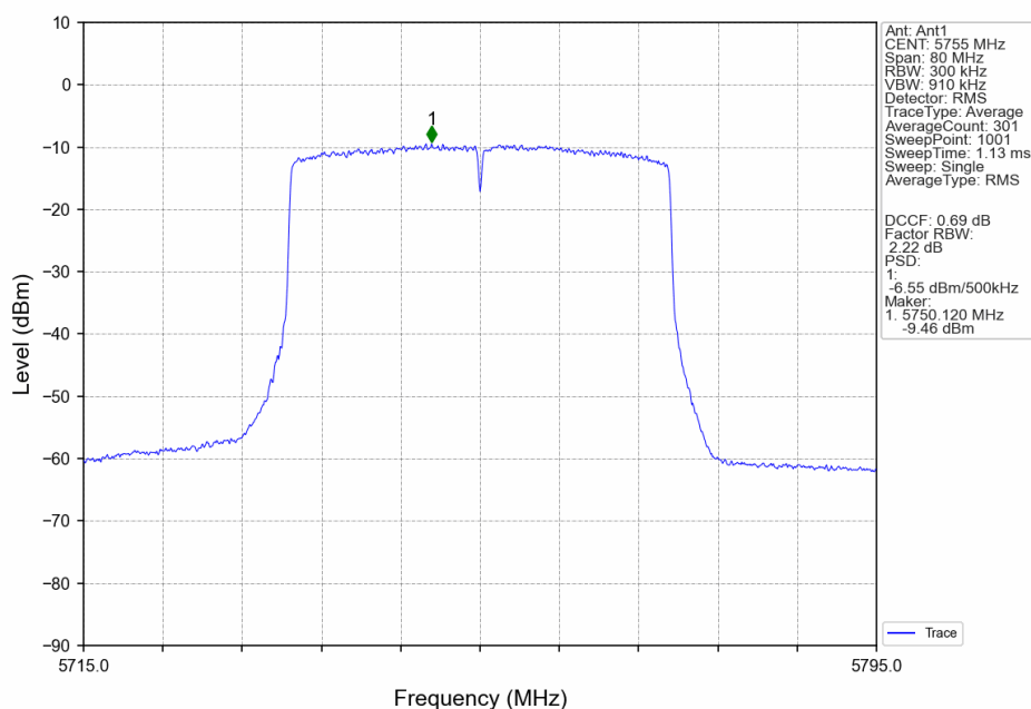
802.11ax(HEW40)_LCH_5755MHz_RU26_Left_Ant1_NTNV
