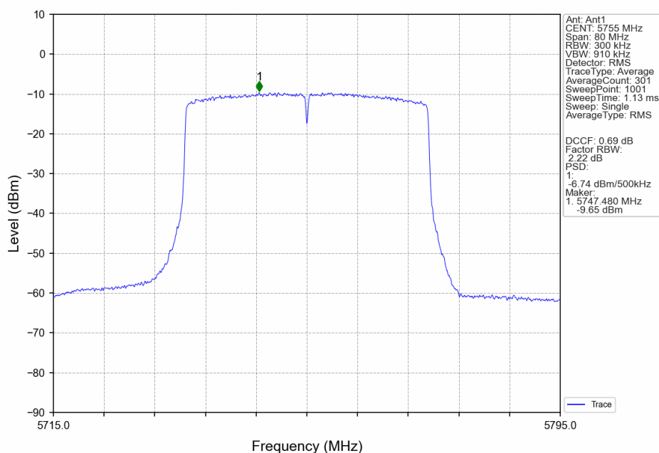
802.11ax(HEW40)_LCH_5755MHz_RU26_Right_Ant1_NTNV
