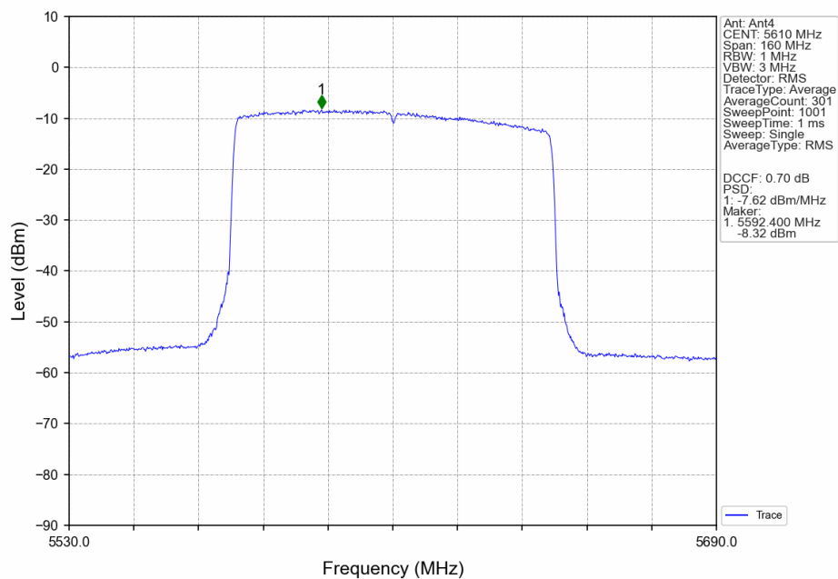
802.11ax(HEW80)_HCH_5610MHz_RU26_Left_Ant4_NTNV
