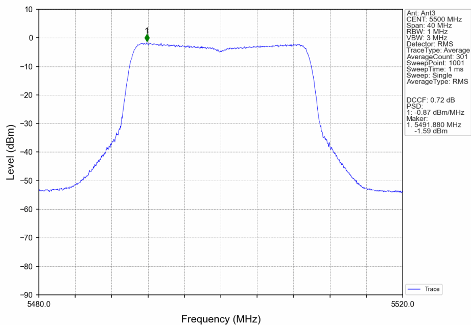
802.11ax(HEW20)_LCH_5500MHz_RU242_Left_Ant3_NTNV
