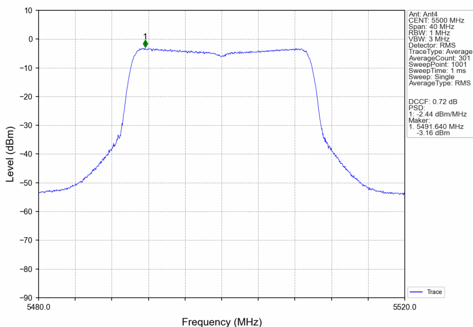
802.11ax(HEW20)_LCH_5500MHz_RU26_Left_Ant4_NTNV
