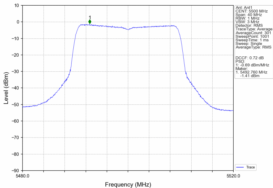
802.11ax(HEW20)_LCH_5500MHz_RU242_Left_Ant1_NTNV
