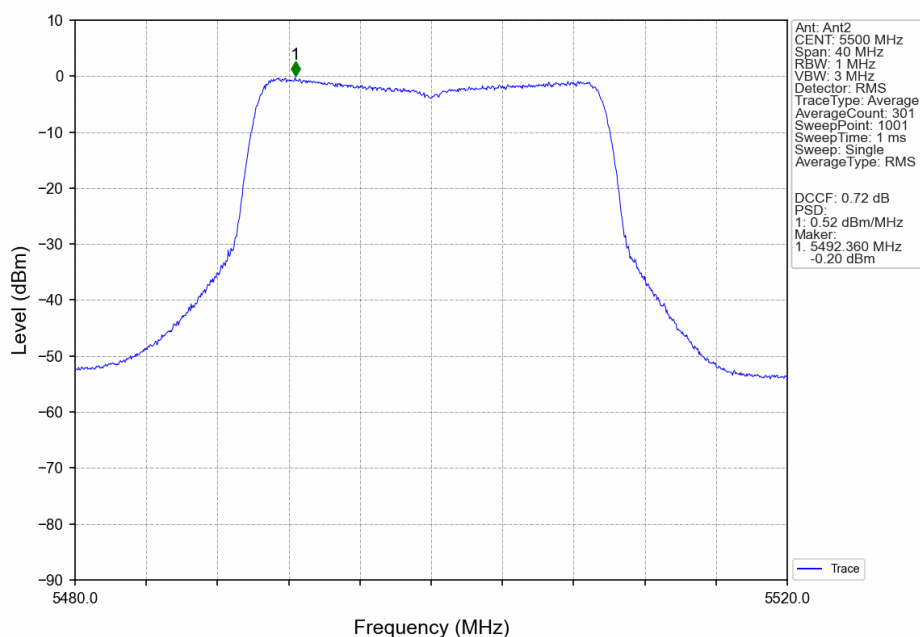
802.11ax(HEW20)_LCH_5500MHz_RU26_Left_Ant2_NTNV
