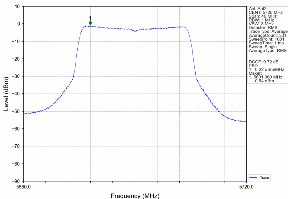
802.11ax(HEW20)_HCH_5700MHz_RU26_Left_Ant2_NTNV
