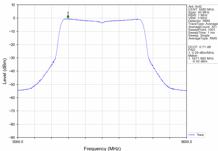
802.11ax(HEW20)_MCH_5580MHz_RU26_Left_Ant2_NTNV
