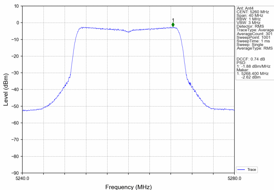
802.11ax(HEW20)_LCH_5260MHz_RU26_Left_Ant4_NTNV
