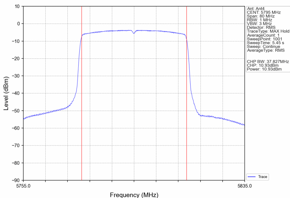
802.11ax(HEW40)_HCH_5795MHz_RU484_Left_Ant4_NTNV
