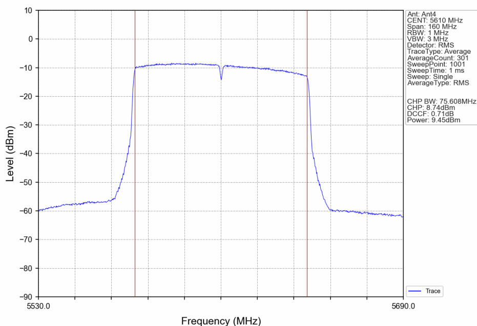
802.11ac(VHT80)_HCH_5610MHz_Ant4_NTNV
